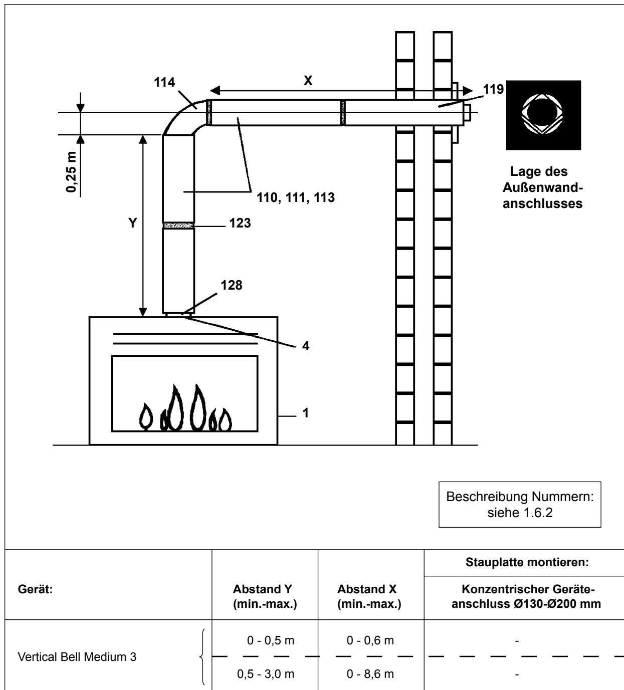
Abbildung 15: Horizontaler Außenwandanschluß
