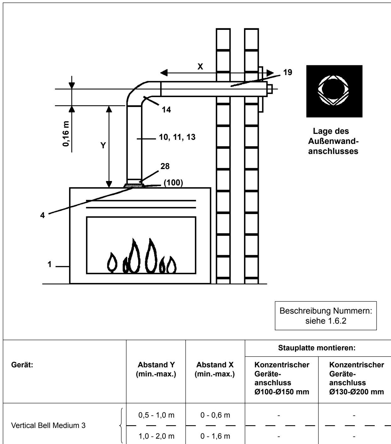
Abbildung 11: Horizontaler Außenwandanschluß
