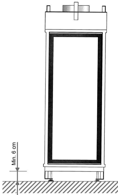
Figura 15: Mínimo 6 cm entre el suelo y la base del aparato
