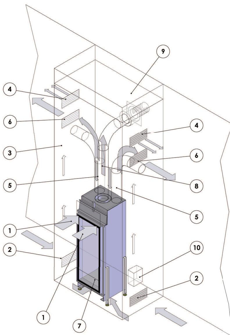
Figura 16: Apparecchio installato in canna fumaria ventilata Scarico orizzontale del gas bruciato / aria di combustione aspirata dal muro.
