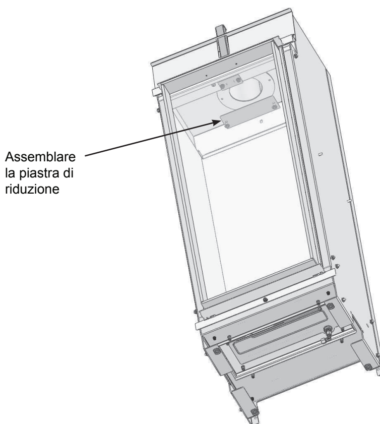
Figura 28: Assemblare la piastra di riduzione
