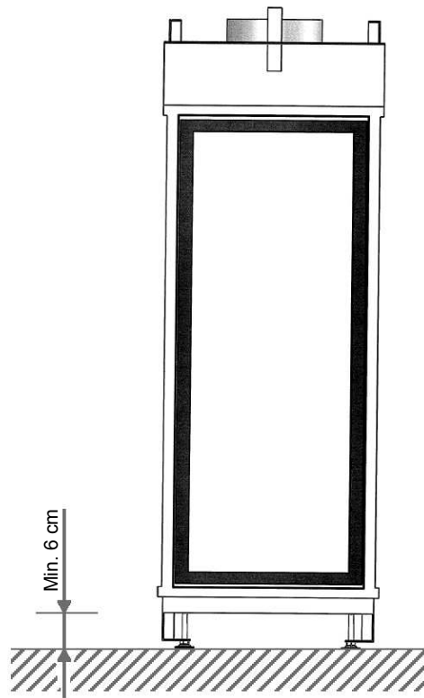
Figuur 15: Minimaal 6 cm ruimte tussen onderzijde toestel en vloer
