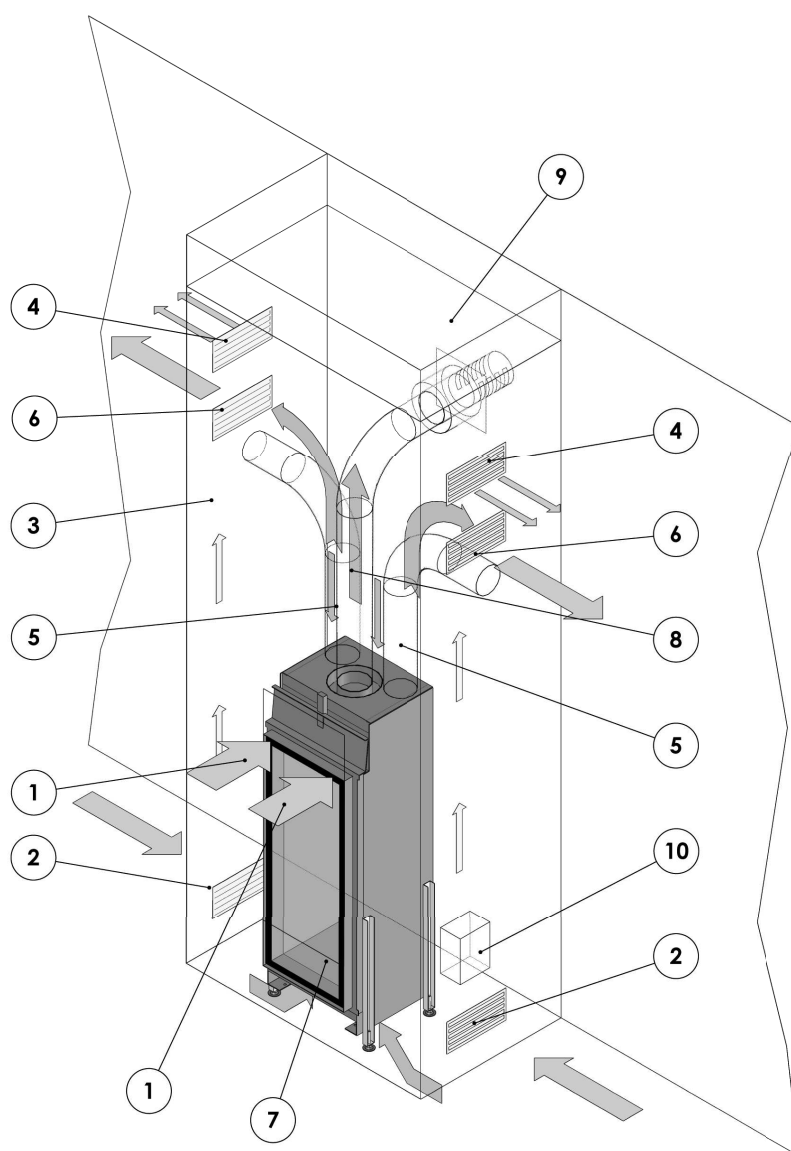
Figuur 16: Toestel ingebouwd in geventileerde schouw Horizontale uitmondung van de rookgasafvoer/verbrandingslucht- toevoer via de muur.
