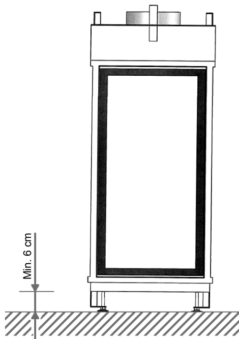
Figura 15: Mínimo 6 cm entre el suelo y la base del aparato
