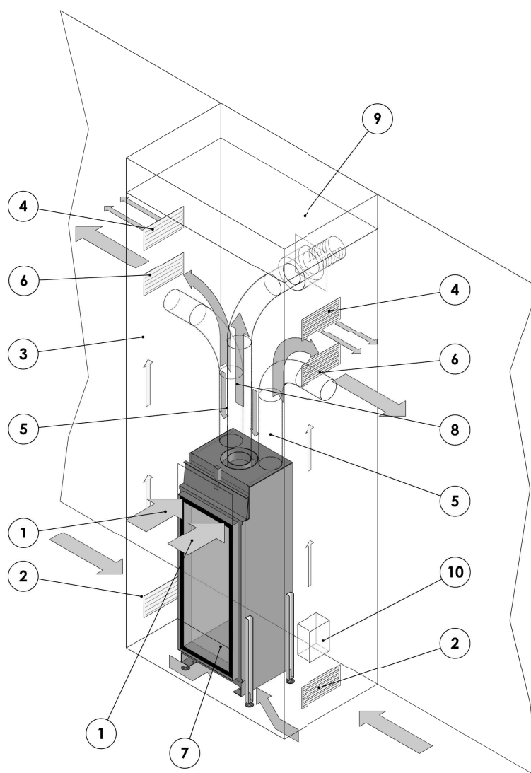
Figura 16: Aparato instalado dentro de una chimenea ventilada Salida horizontal de evacuación de gases de combustión / aire de combustión suministrado a través de la pared.
