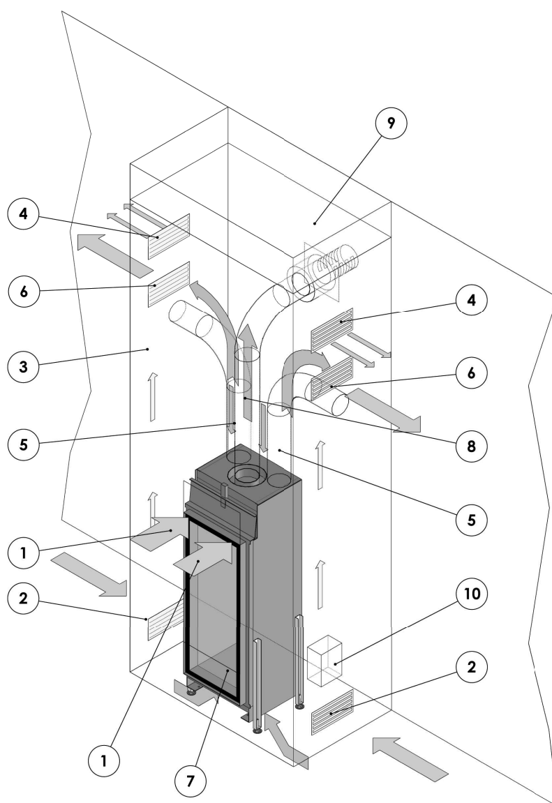
Figure 16: Appareil installé dans une cheminée ventilée Sortie horizontale de l'évacuation des gaz de combustion / l'alimentation en air de combustion par le biais du mur.
