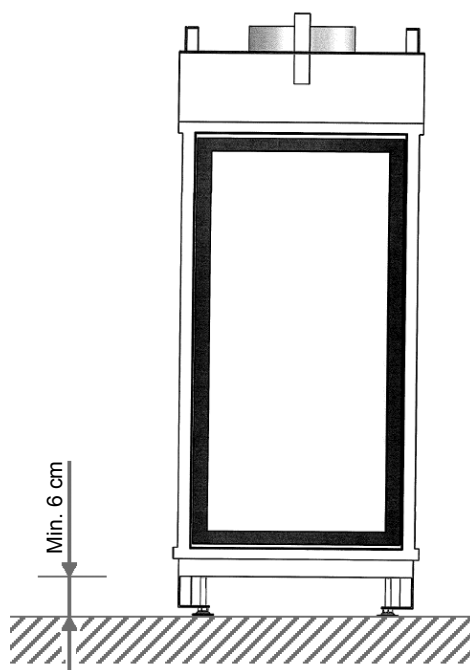
Figure 15: 6 cm au minimum entre le sol et l'appareil en bas
