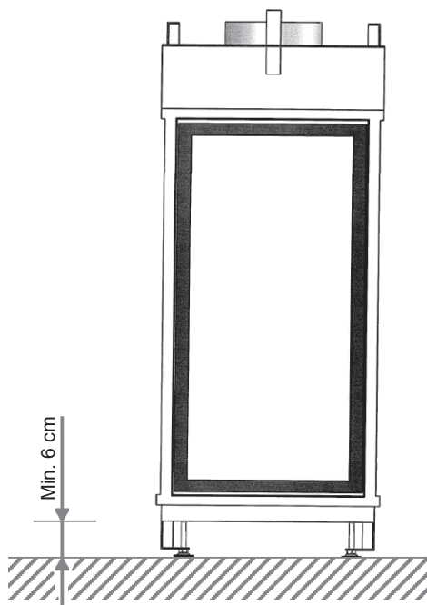
Figura 15: Deve essere mantenuto uno spazio di almeno 6 cm tra la base dell'apparecchio e il pavimento.
