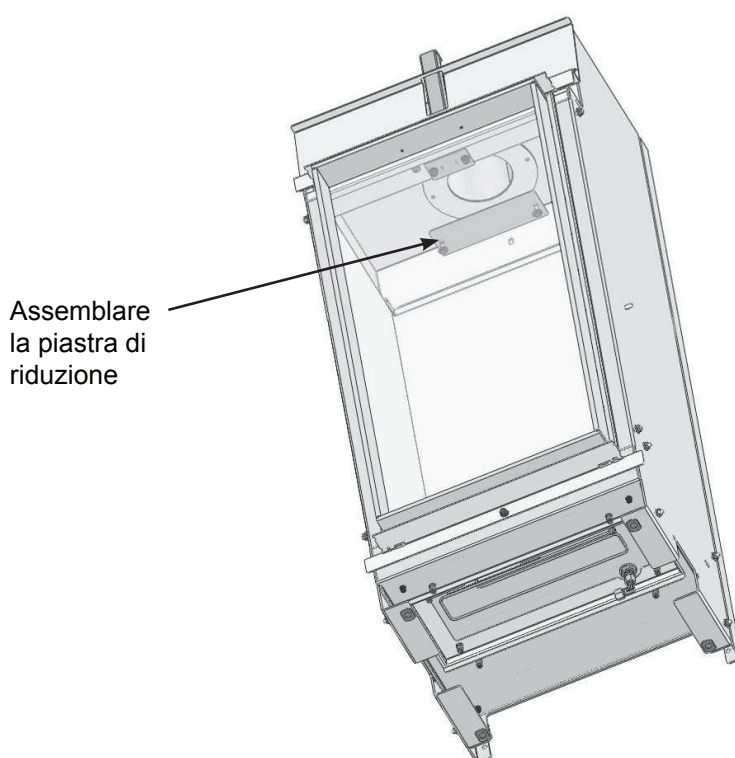
Figura 28: Assemblare la piastra di riduzione
