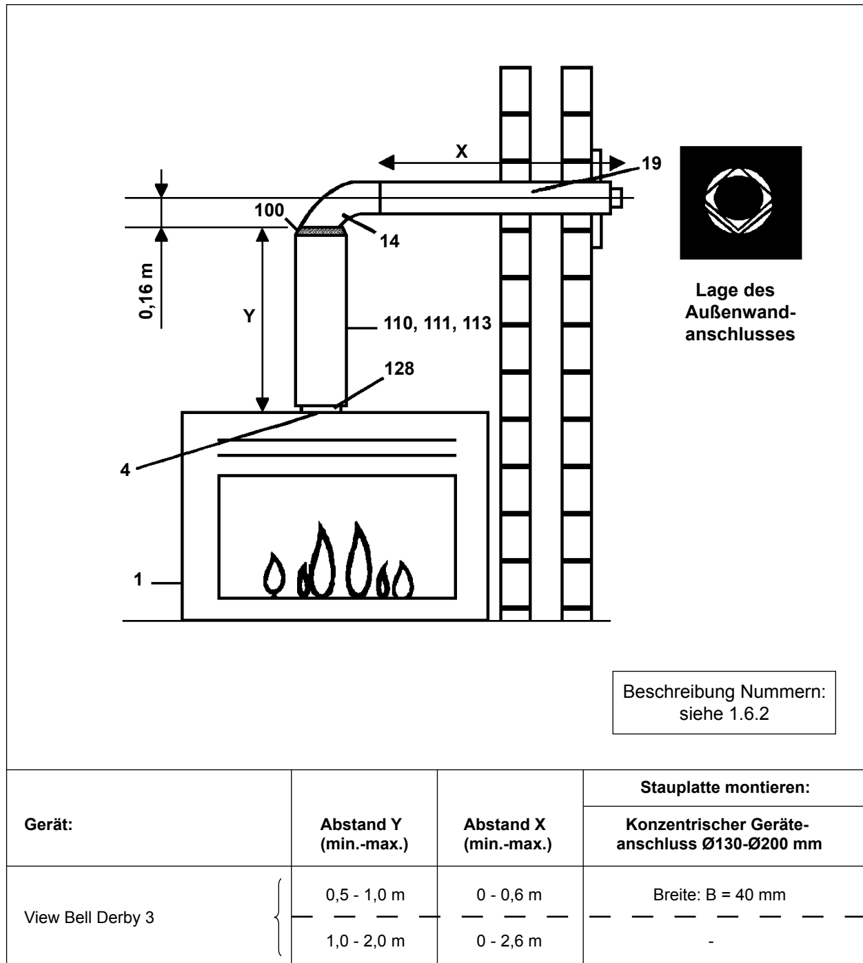
Abbildung 12: Horizontaler Außenwandanschluß
