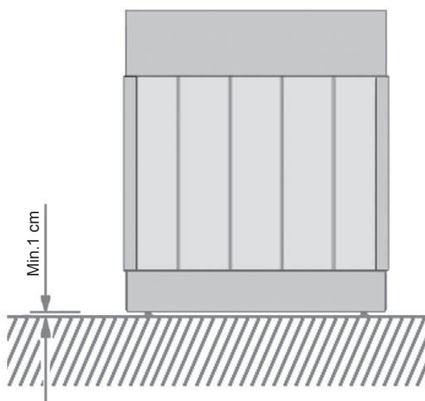
Figura 15: Mínimo 1 cm entre el suelo y la base del aparato
