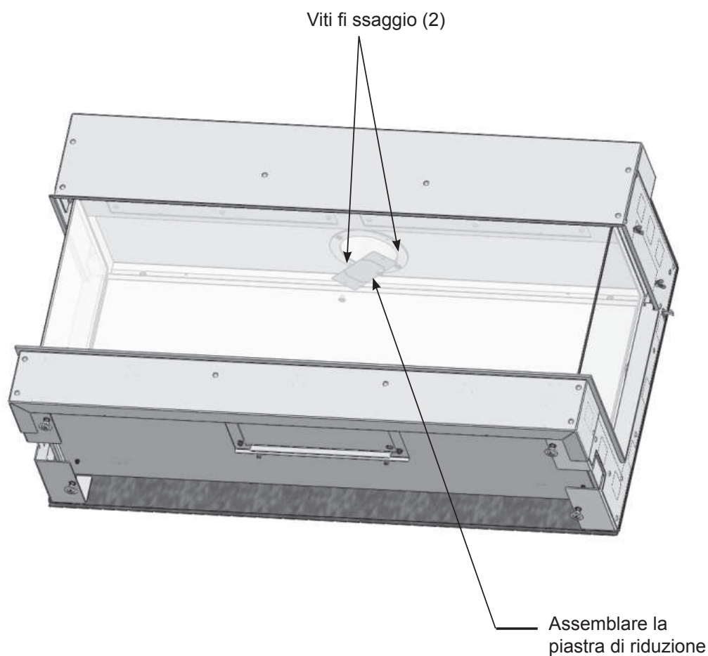
Figura 28: Assemblare la piastra di riduzione
