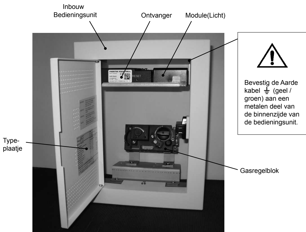
Figuur 23D: Inbouw bedieningsunit Positie Ontvanger, Module(Licht) en Gasregelblok (Componenten zijn op de foto nog niet elektrisch aangesloten!)
