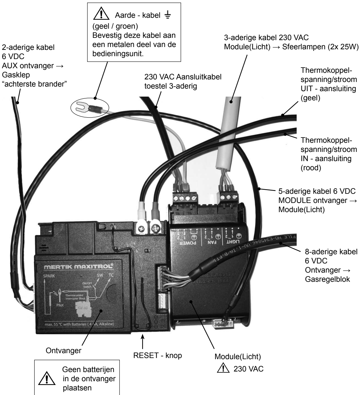
Figuur 23B: Elektrische aansluitingen Ontvanger en Module(Licht)
