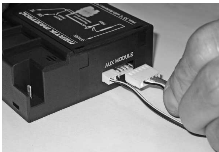
Figuur 23C: Aansluiten 5-aderige kabel 6VDC op MODULE aansluiting van de ontvanger
