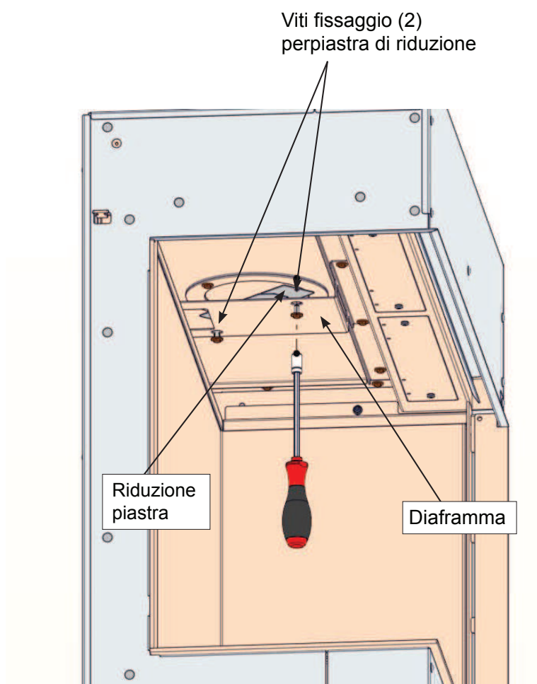
Figura 28: Assemblare la piastra di riduzione
