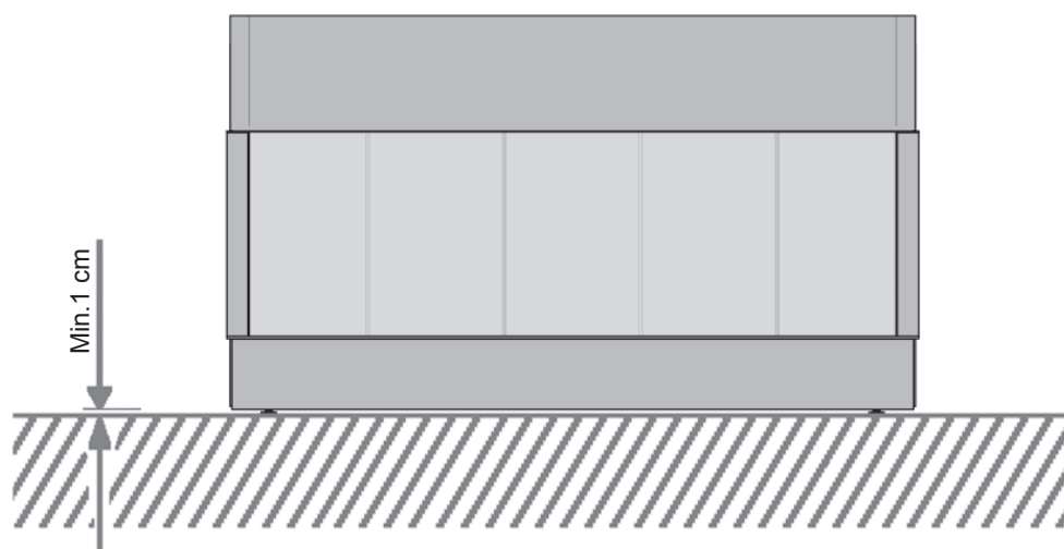
Figura 15: Deve essere mantenuto uno spazio di almeno 1 cm tra la base dell'apparecchio e il pavimento.
