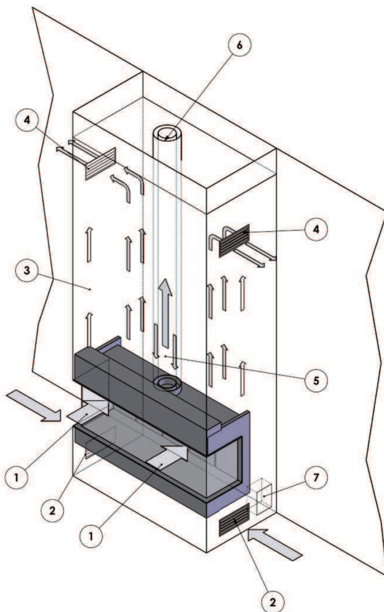
Figura 17: Apparecchio installata in canna fumaria ventilata Scarico verticale del gas bruciato / aria di combustione aspirata dal tetto. Montato senza kit di convezione
