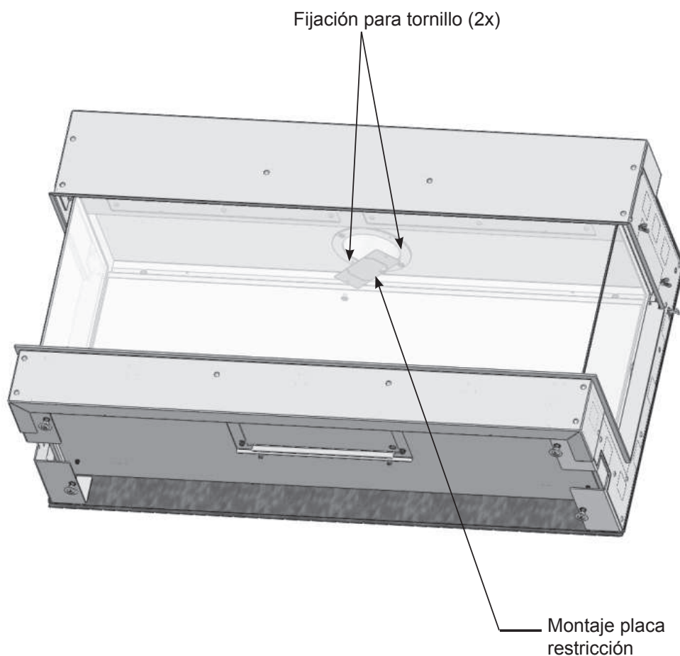
Figura 28: Colocación de la placa de restricción
