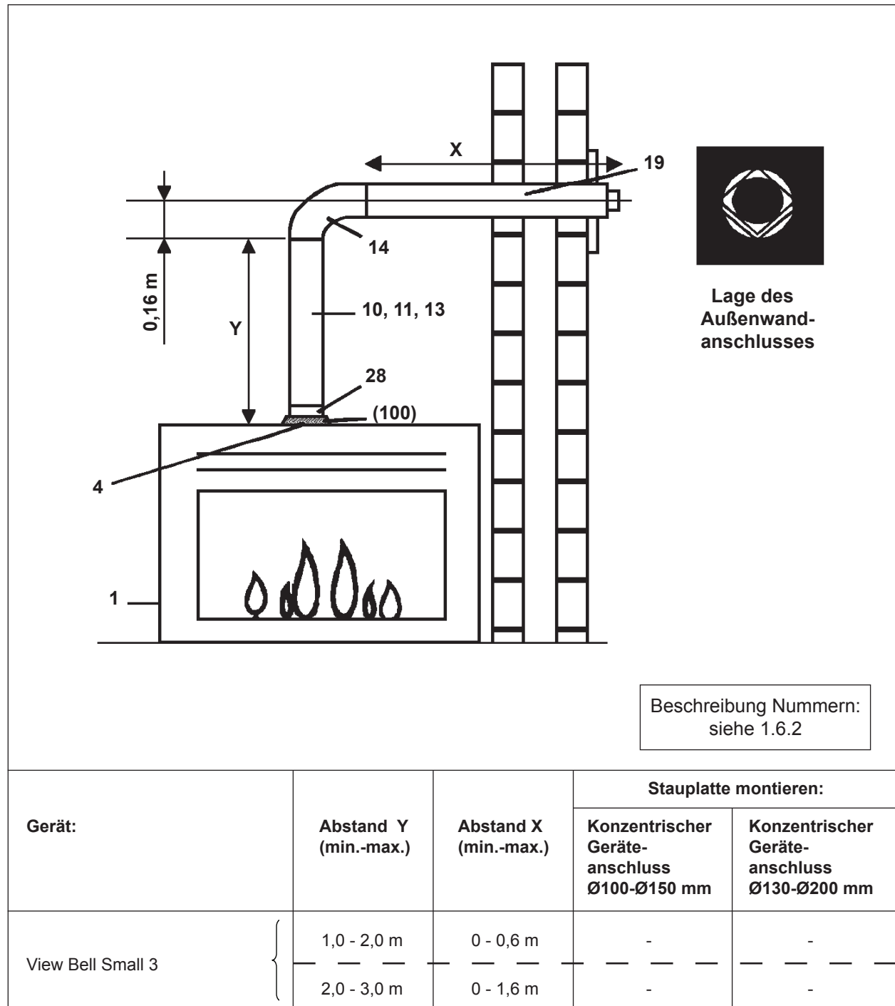
Abbildung 11: Horizontaler Außenwandanschluß
