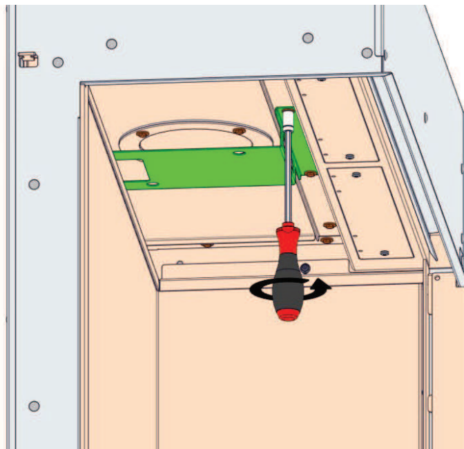
Abbildung 30: Entfernung der Umlenkplatte
