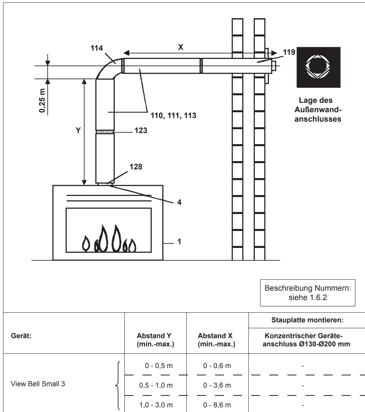
Abbildung 15: Horizontaler Außenwandanschluß
