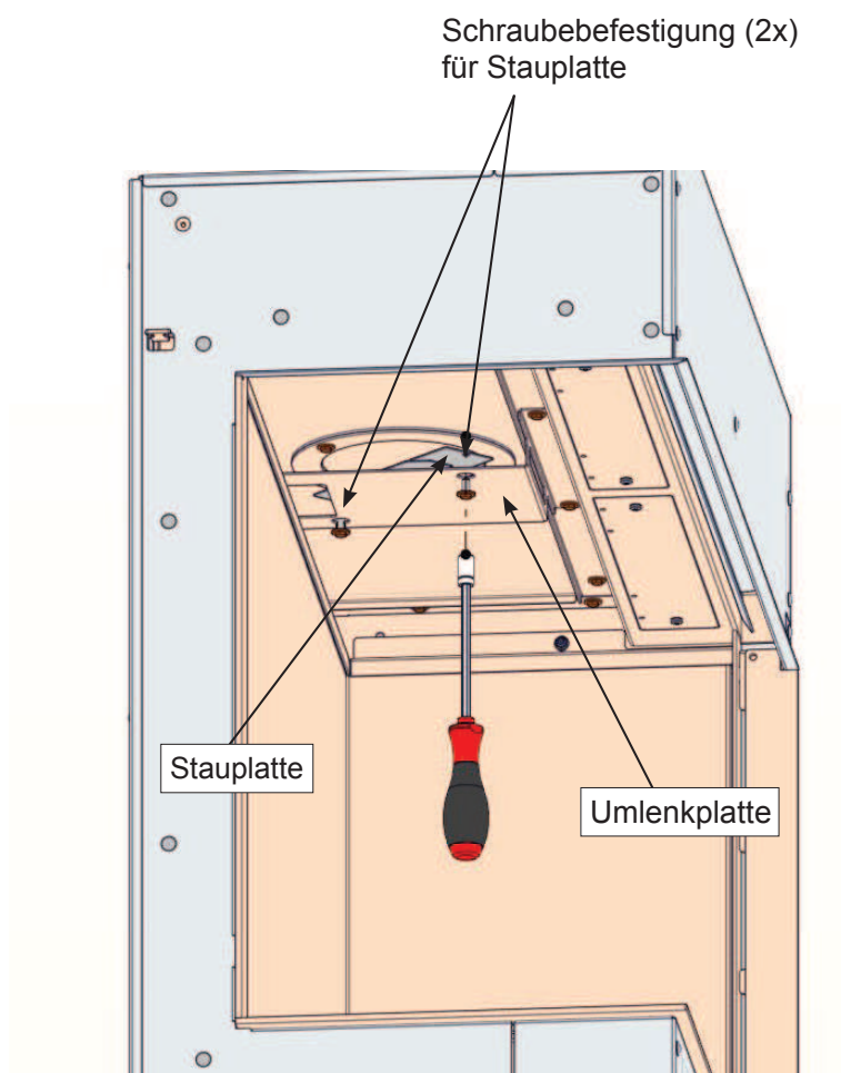
Abbildung 29: Montage Stauplatte
