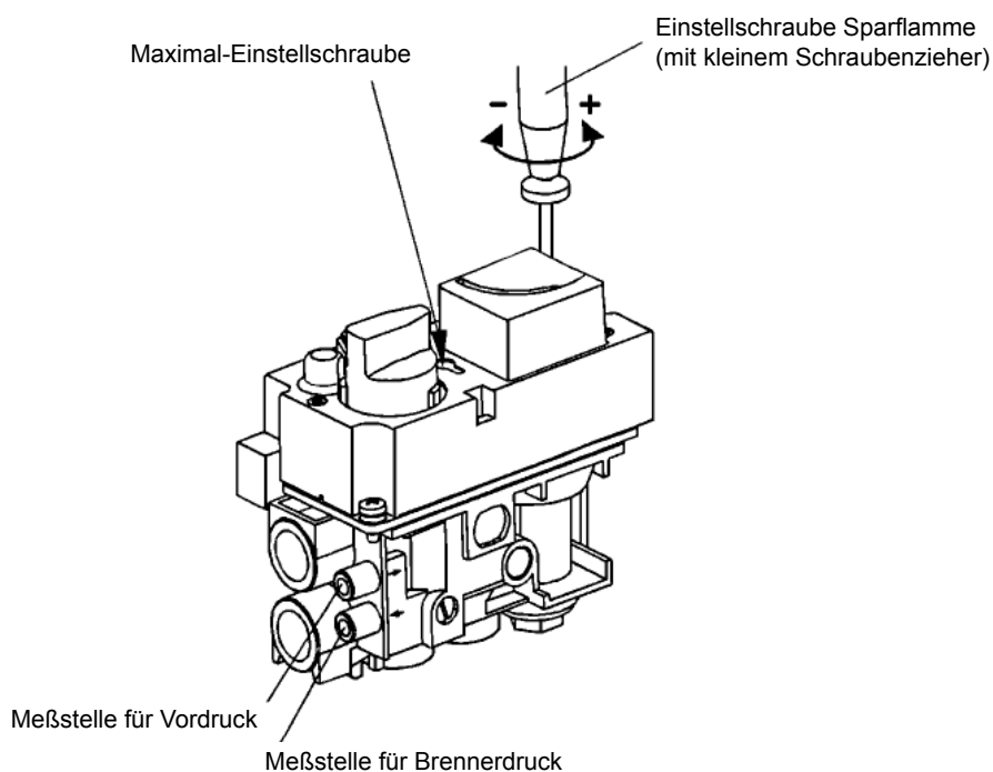
Abbildung 1: Gasregelblock Fernbedienung (Gerät mit Bedienungseinheit)
