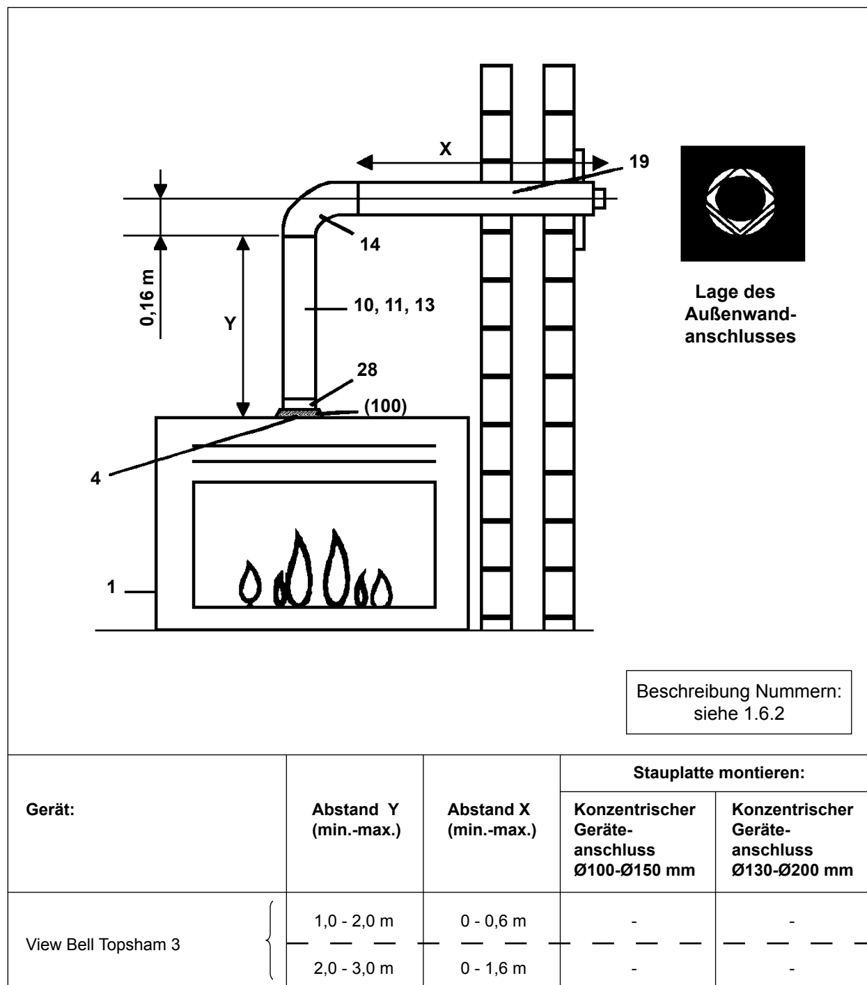
Abbildung 11: Horizontaler Außenwandanschluß
