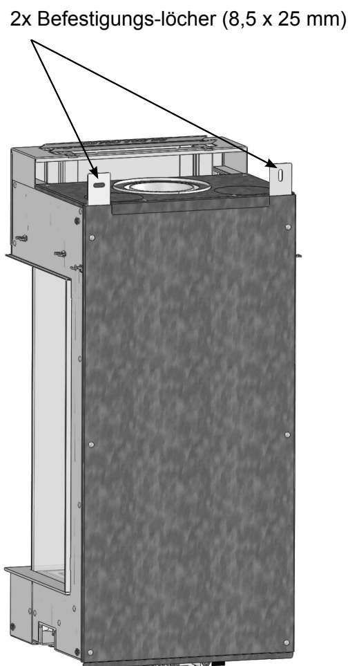
Abbildung 22: Befestigungs-löcher (2x) Hinterseite Hängekamin
