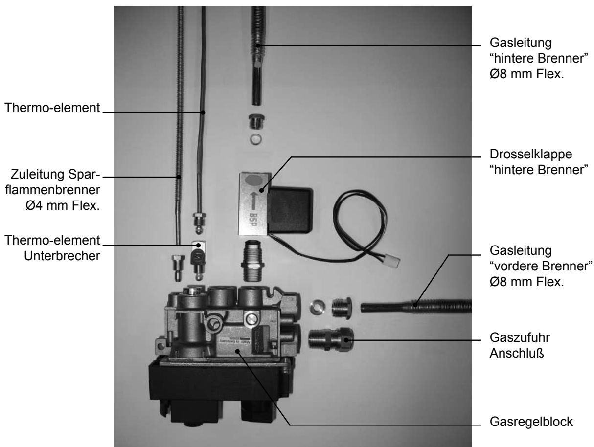
Abbildung 24: Gasregelblock und Drosselklappe: Gas und Thermo-element Anschluß
