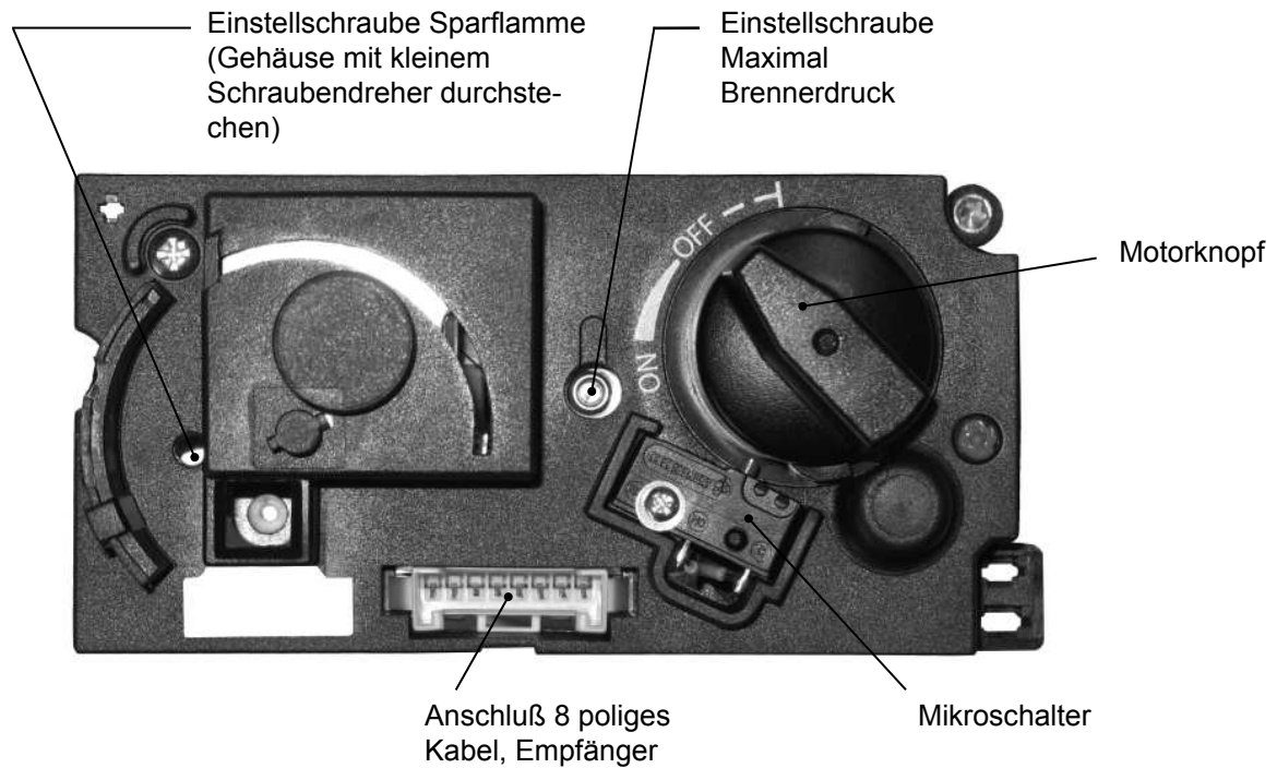
Abbildung 25: Gasregelblock - Vorderseite
