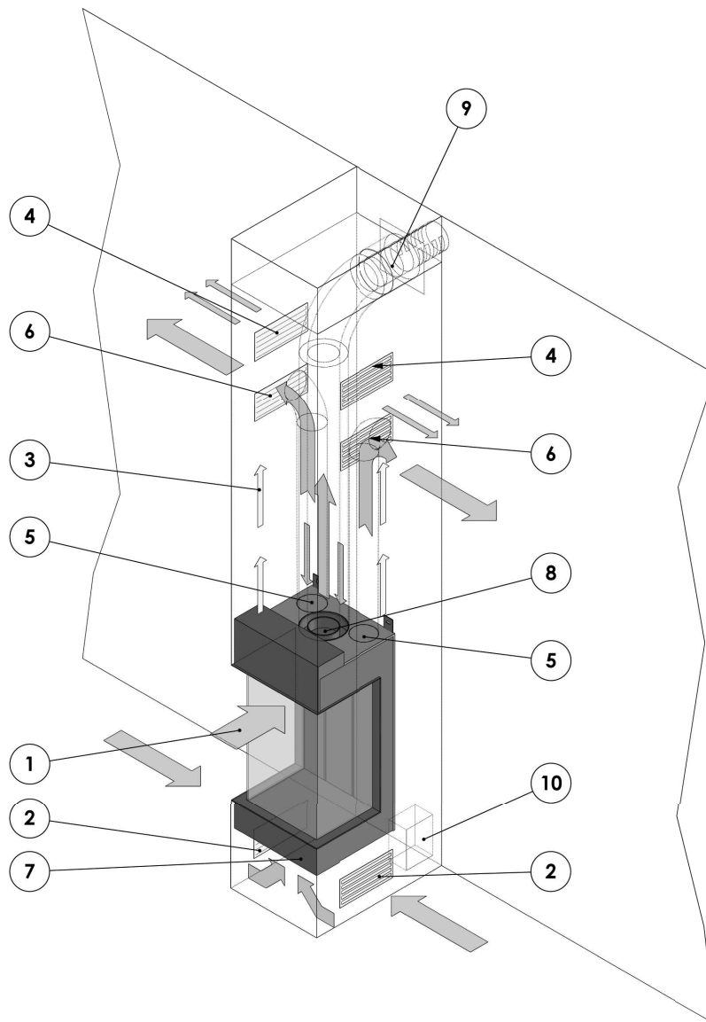
Abbildung 17: EINBAUKAMIN: Gerät in belüfteten Kaminmantel eingebaut Horizontaler Abzug der Zu-/Abluft über die Wand Optionen/Zubehör:
