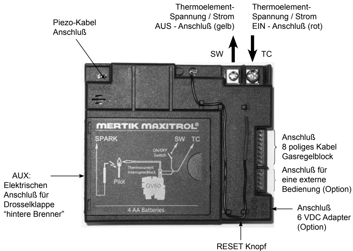
Abbildung 27: Empfänger - Oberseite
