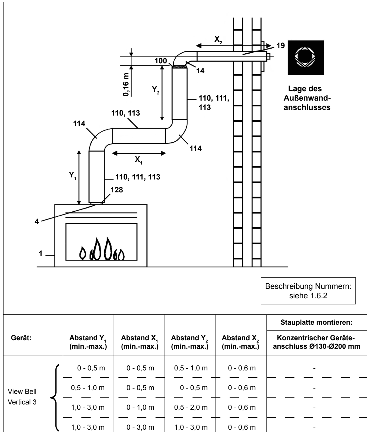
Abbildung 14: Horizontaler Außenwandanschluß
