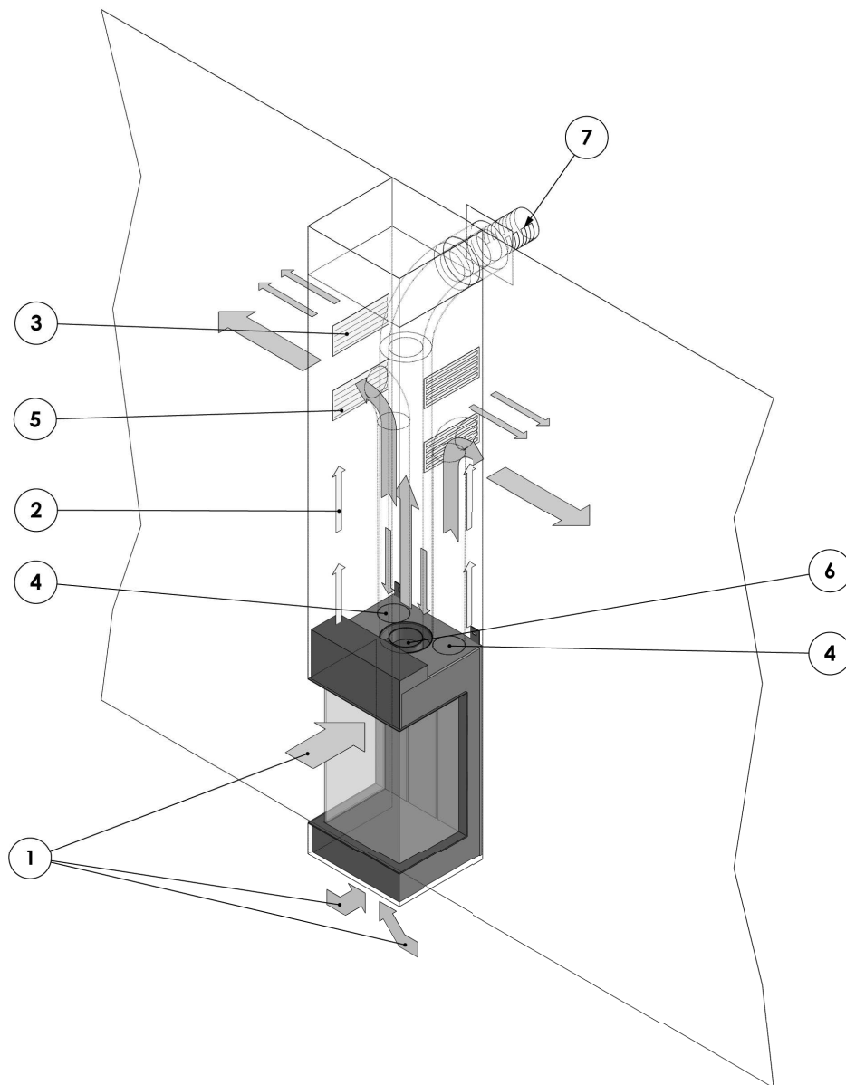
Abbildung 19: HÄNGEKAMIN:
