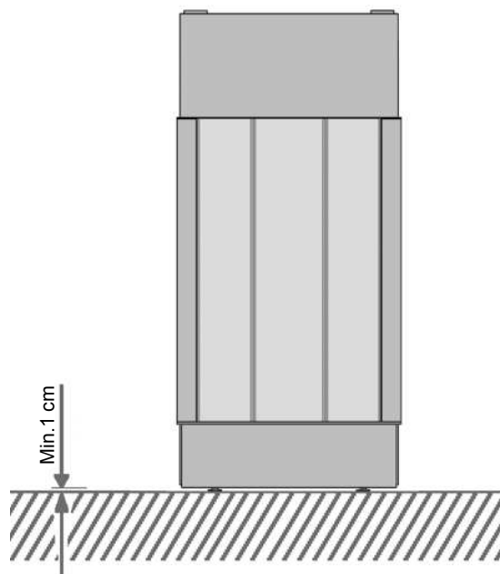
Abbildung 16: Minimal 1 cm Spiel zwischen die Unterseite des Geräts und dem Boden
