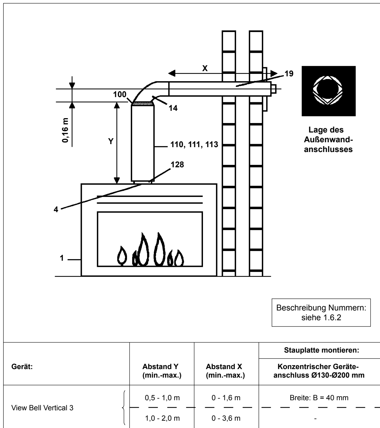
Abbildung 12: Horizontaler Außenwandanschluß
