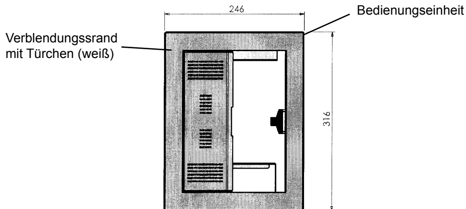
Abbildung 23: Bedienungseinheit
