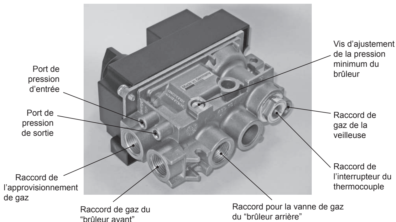
Figure 23: Bloc de régulateur du gaz - Arrière
