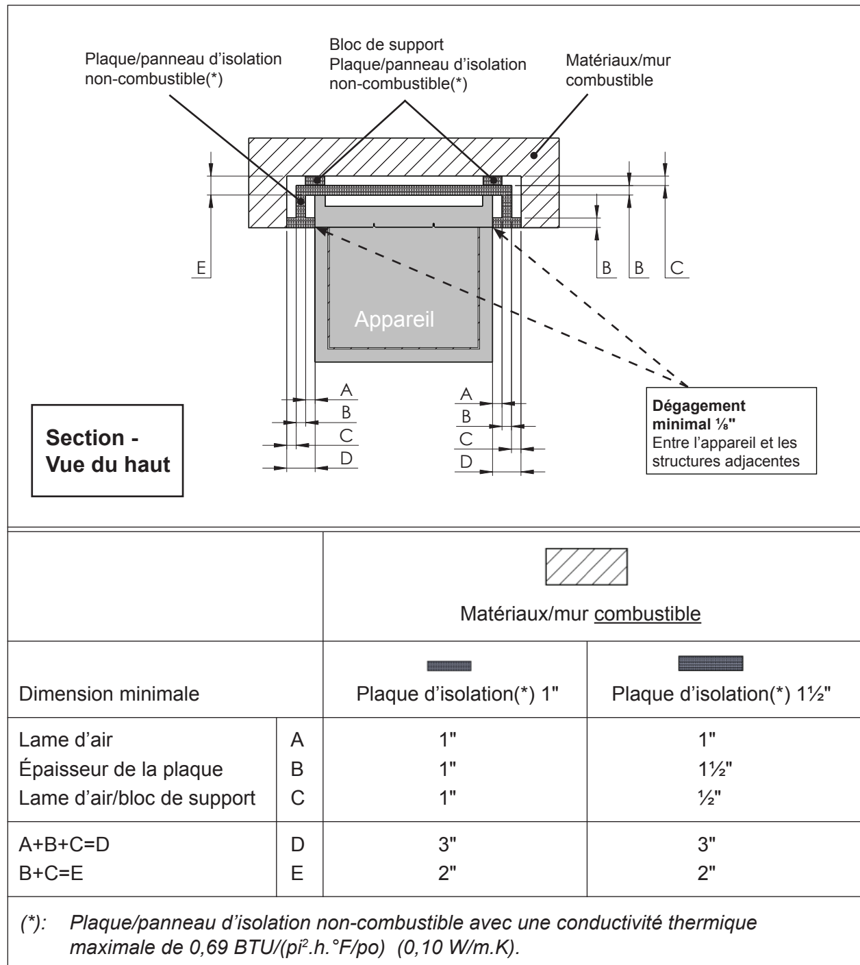
Figure 1: Dégagement jusqu'aux côtés combustibles et épaisseur minimale requise pour la plaque/panneau(*) non-combustible
