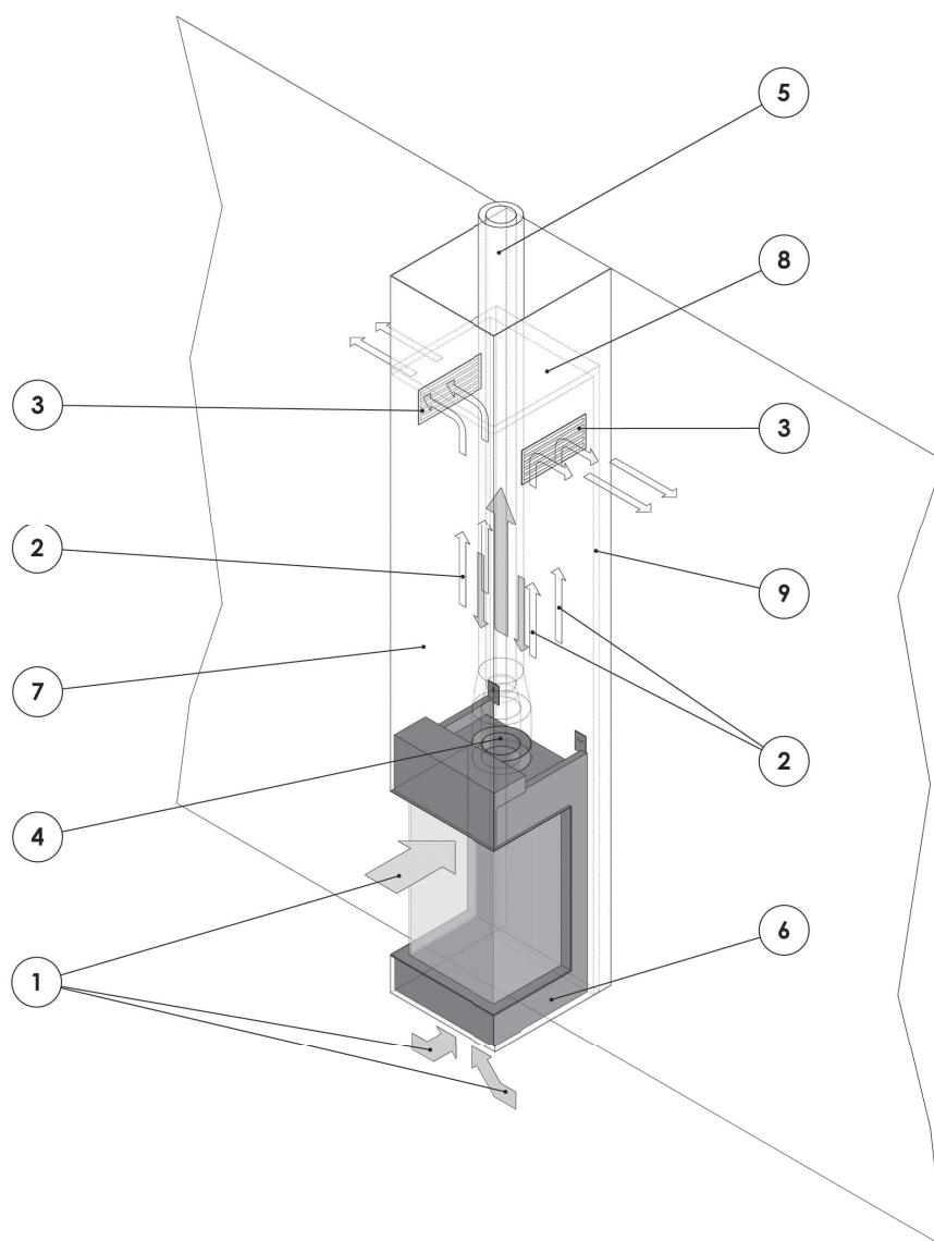
Figure 18: APPAREIL MURALE: Appareil avec manteau ventilé Terminaison verticale d'évacuation de la fumée/source d'air de combustion au travers du toit.
