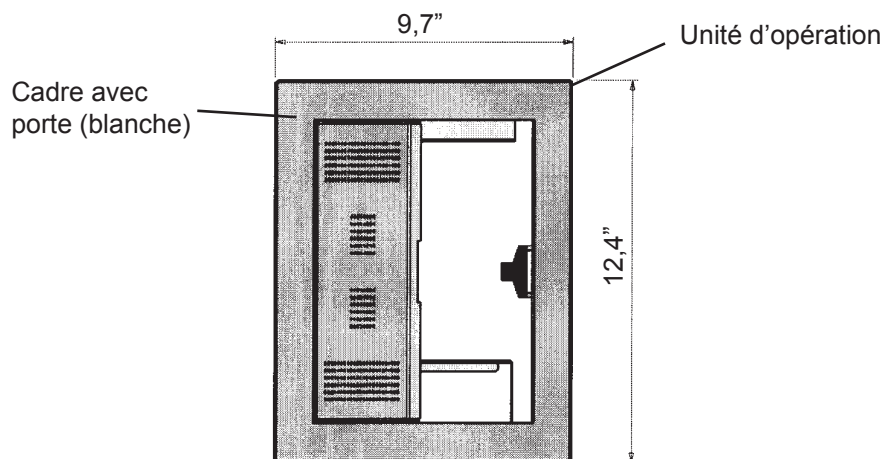
Figure 20: Unité d'opération
