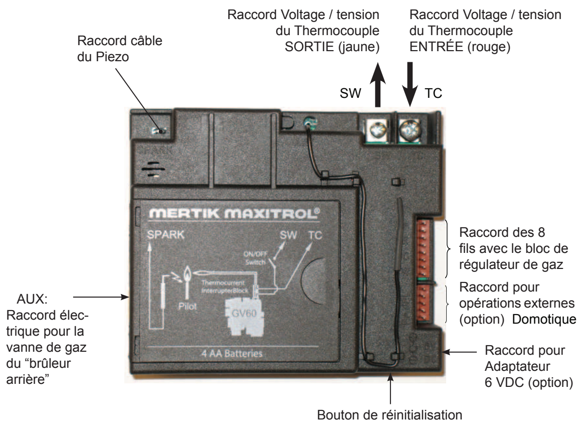
Figure 24: Récepteur - vue du dessus
