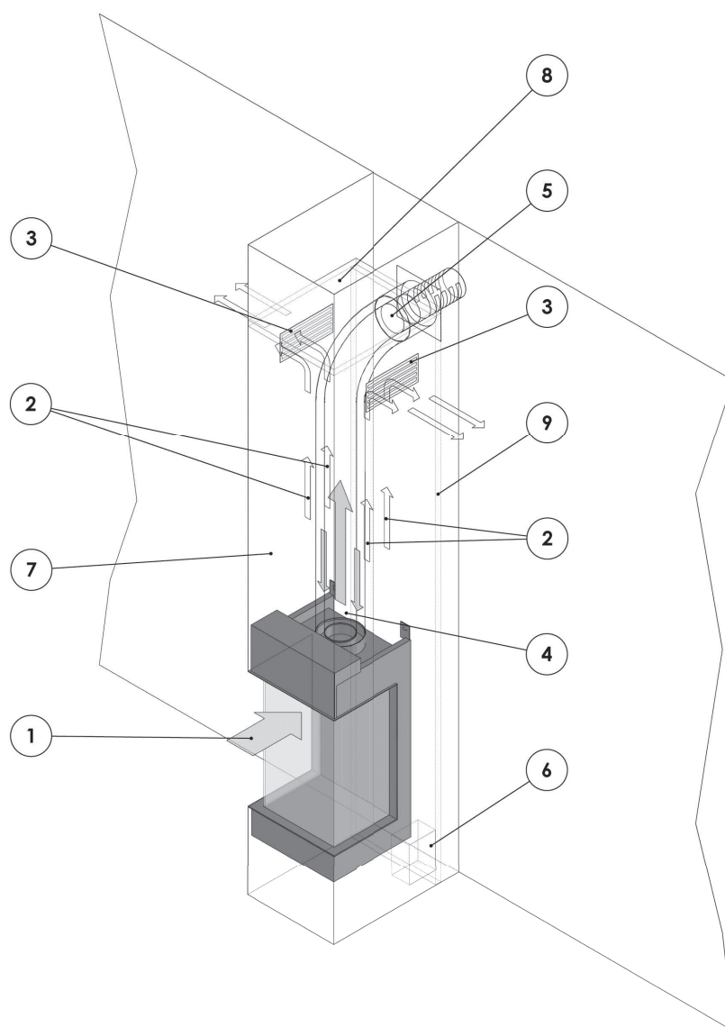
Figure 15: Appareil installé dans le manteau d'une cheminée ventilée/Enchassement Terminaison horizontale d'évacuation de la fumée/source d'air de combustion au travers du mur.
