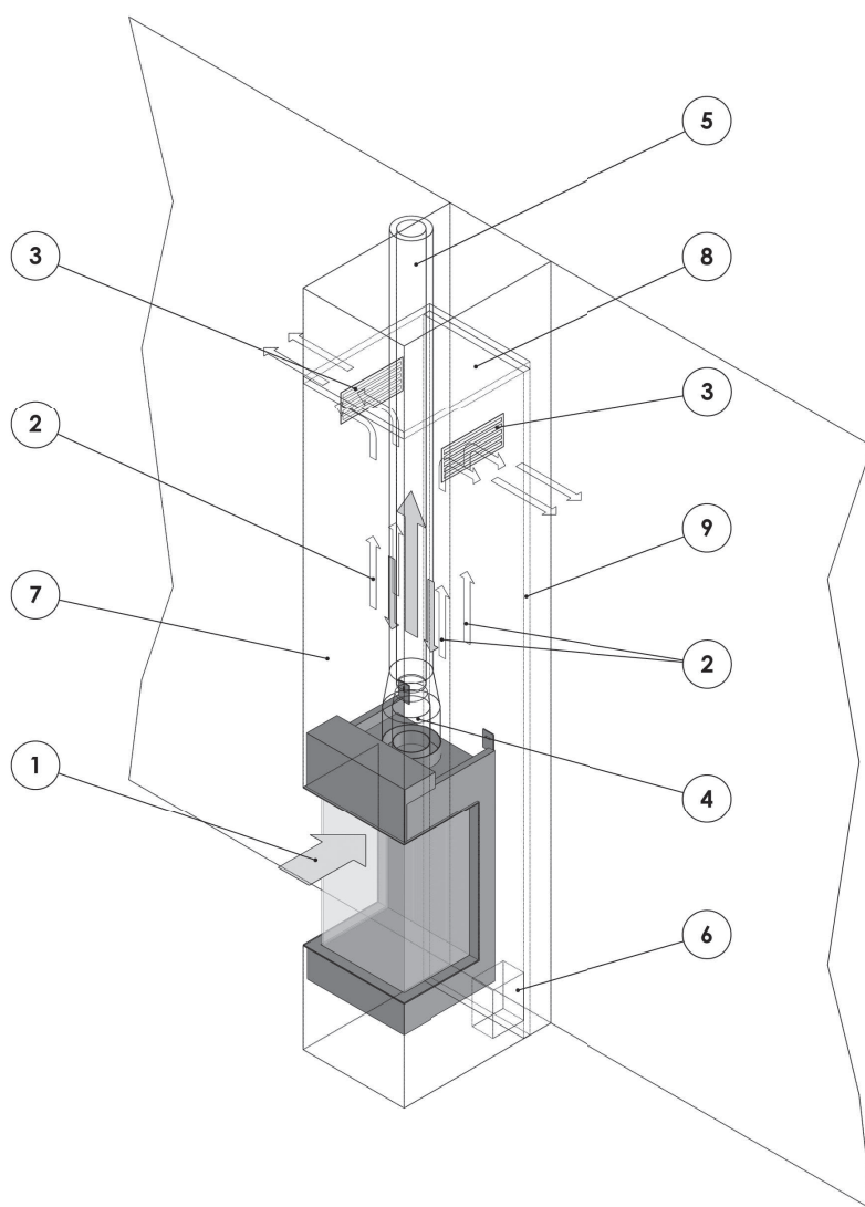
Figure 16: Appareil installé dans le manteau d'une cheminée ventilée/Enchassement Terminaison verticale d'évacuation de la fumée / source d'air de combustion au travers du toit.
