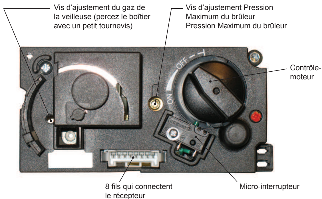
Figure 22: Bloc de régulateur du gaz - Avant
