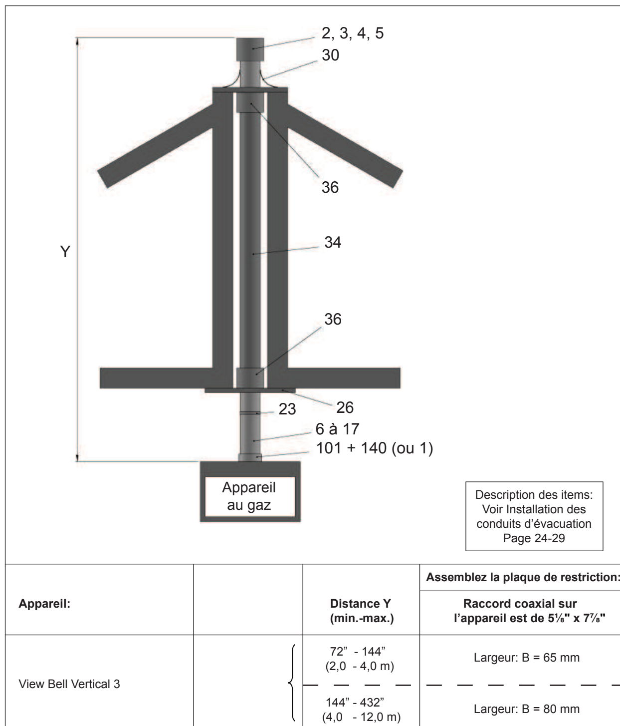
Figure 11: Terminaison verticale utilisant une cheminée munie d'une doublure existante (Flexible 4" et/ou rigide 4" x 6 5 / 8 " )
