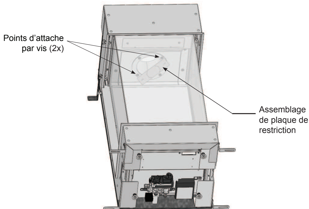
Figure 28: Mise en place de la plaque de restriction
