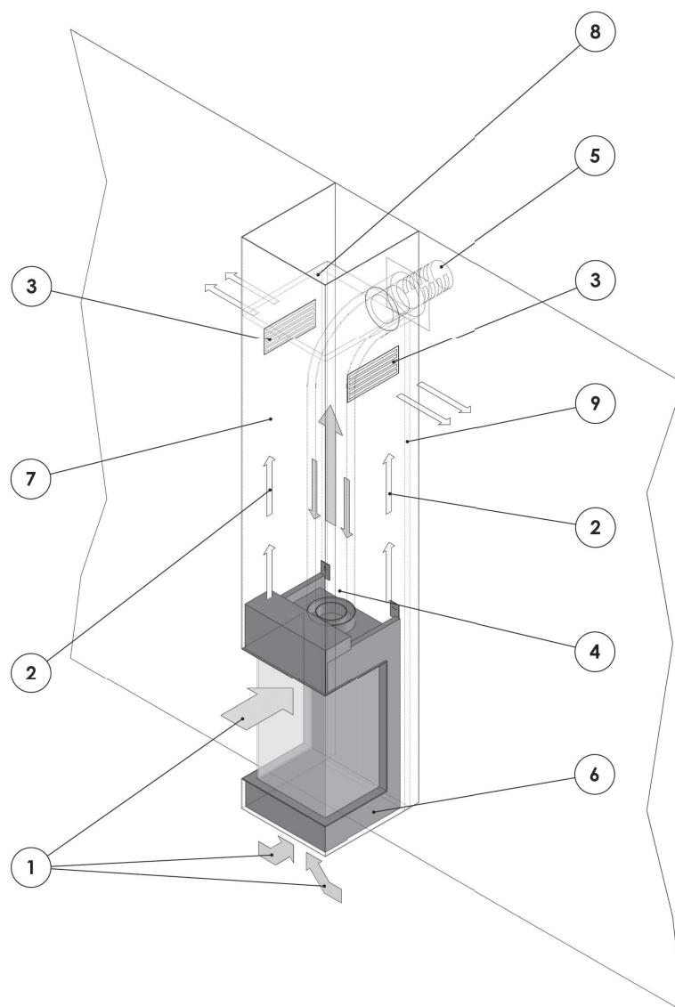
Figure 17: APPAREIL MURALE: Appareil avec manteau ventilé Terminaison horizontale d'évacuation de la fumée/source d'air de combustion au travers du mur.
