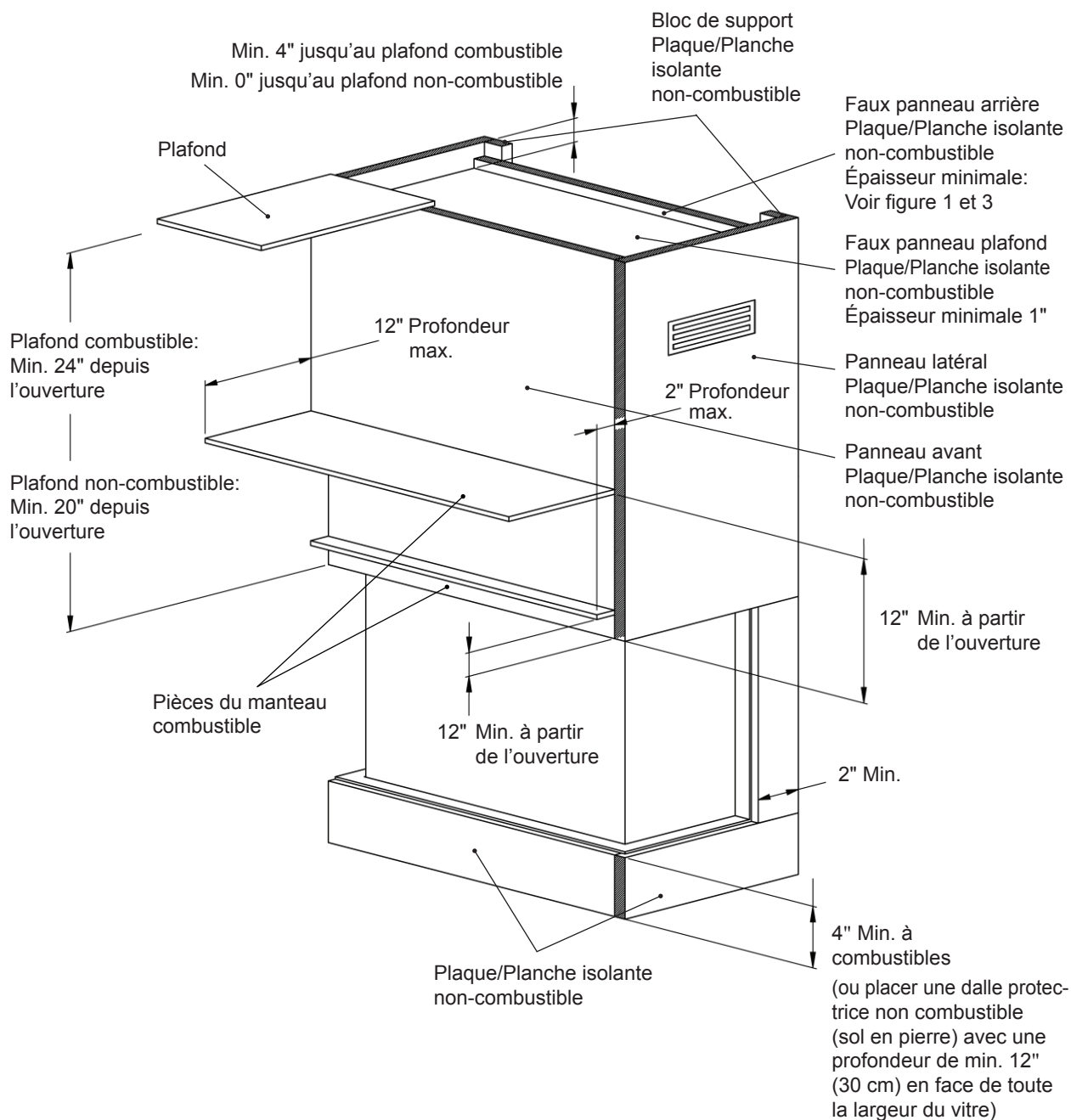
Figure 5: Dégagements du manteau
