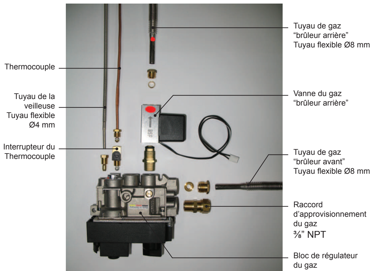
Figure 21: Bloc de régulateur de gaz et vanne de gaz: Raccords du gaz et du thermocouple
