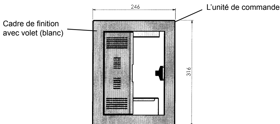
Figure 22: L'unité de commande
