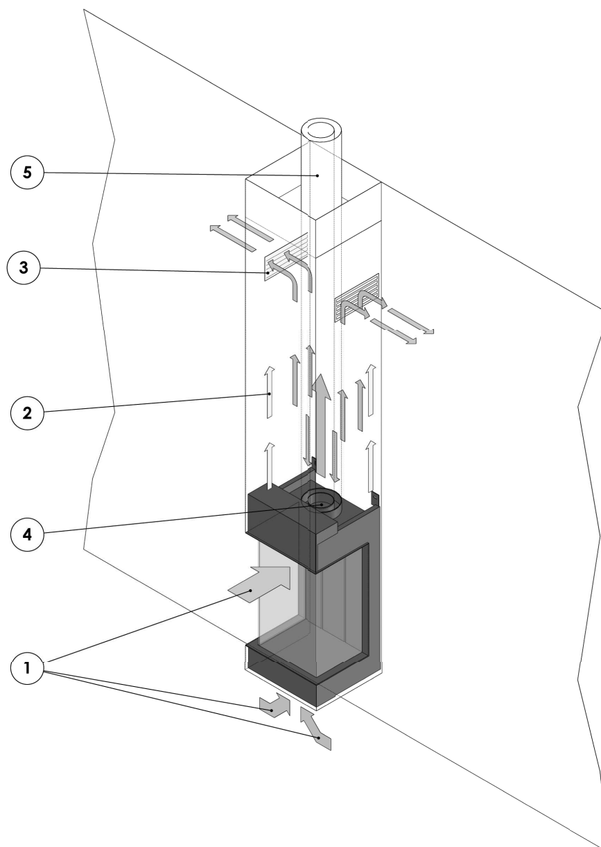
Figure 19: FOYER SUSPENDU: Appareil installé avec une voûte ventilée Sortie verticale de l'évacuation des gaz de combustion / l'alimentation en air de combustion par le biais du toit. Application sans kit de convection.
