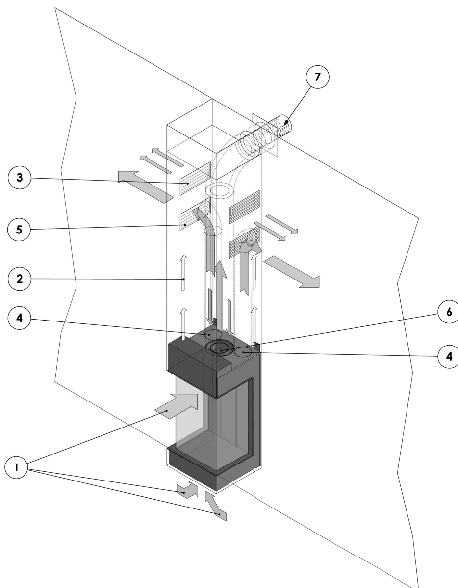
Figure 18: FOYER SUSPENDU: Appareil installé avec une voûte ventilée Sortie horizontale de l'évacuation des gaz de combustion / l'alimentation en air de combustion par le biais du mur. Doté des options/accessoires: • kit de convection (= manteau de convection et 1x jeu de convection)
