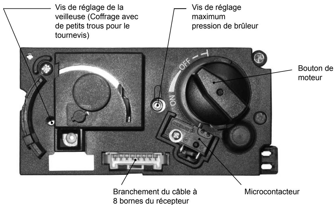
Figure 24: Bloc de réglage du gaz - Devant
