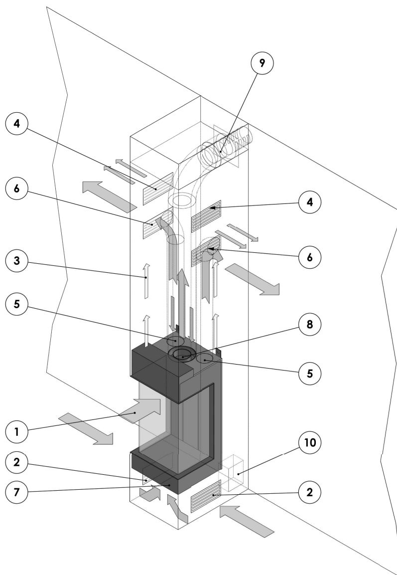
Figure 16: FOYER ENCASTRER: Appareil installé dans une cheminée ventilée Sortie horizontale de l'évacuation des gaz de combustion / l'alimentation en air de combustion par le biais du mur. Doté des options/accessoires: • kit de convection (= manteau de convection et 1x jeu de convection)
