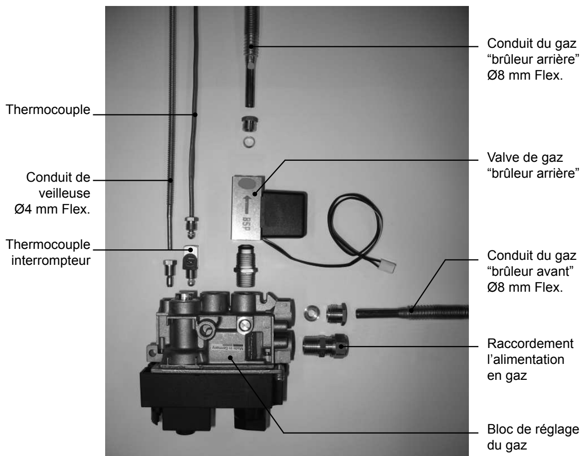
Figure 23: Bloc de réglage du gaz et valve de gaz: Raccordements de gaz et le thermocouple
