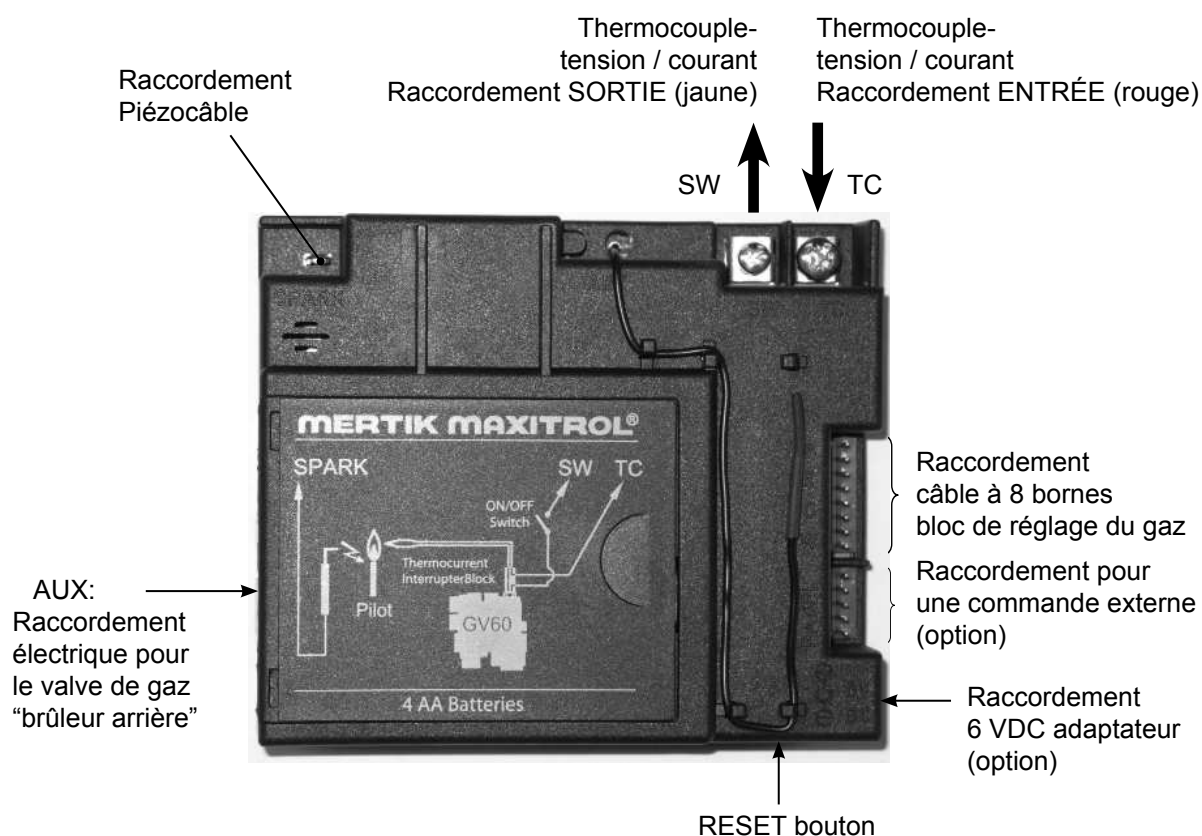
Figure 26: Récepteur - Dessus
