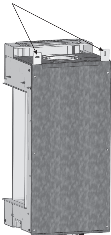
Figura 21: Fori di montaggio (2) Apparecchio con muro posteriore
