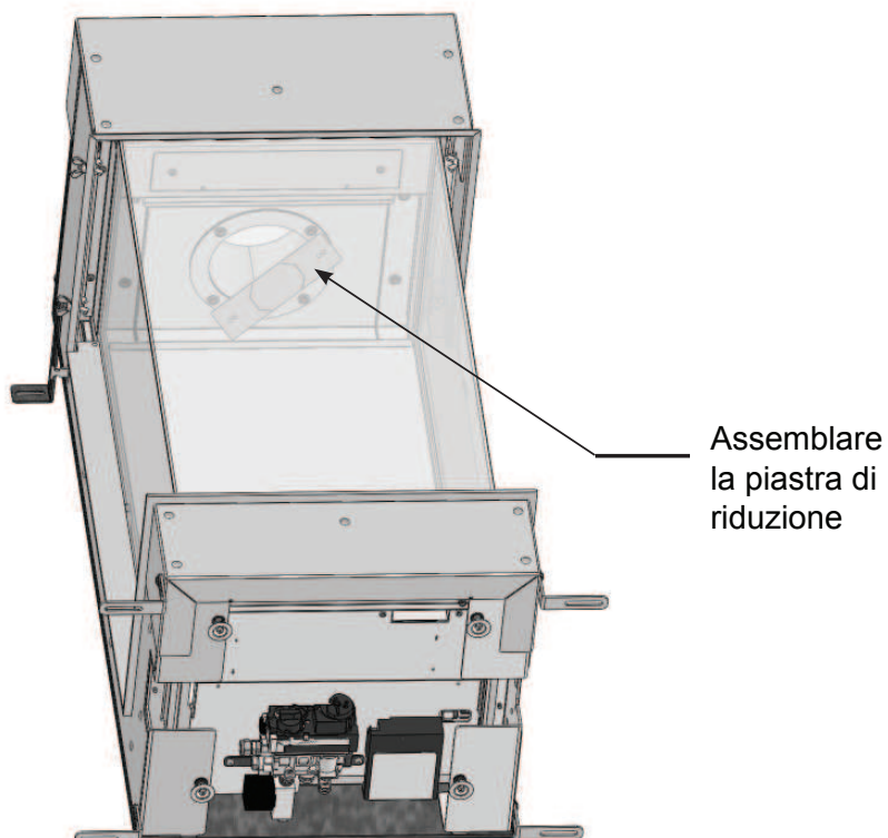
Figura 32: Assemblare la piastra di riduzione
