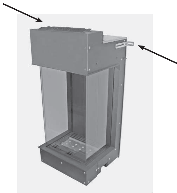
Figura 20: Staffe di montaggio (2)
