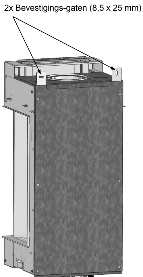
Figuur 21: Bevestigingsgaten (2x) Achterzijde Hang-Haard
