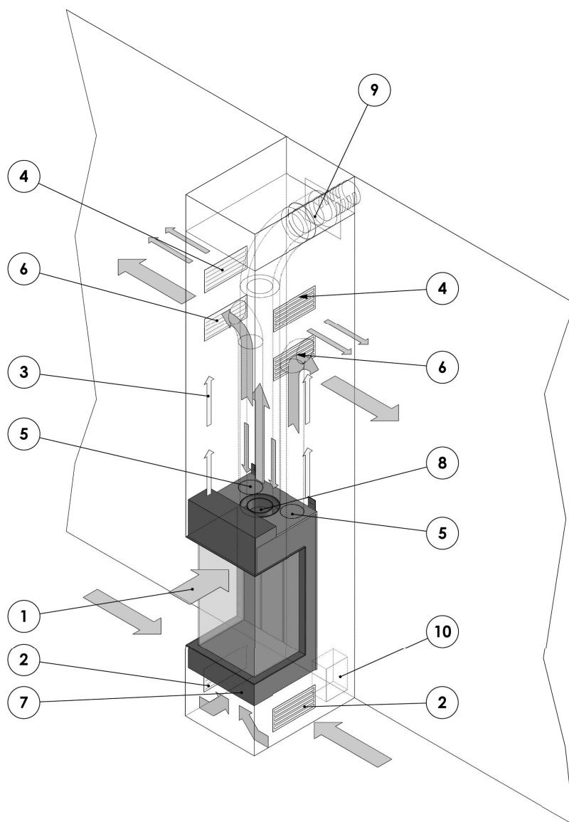
Figuur 16: INBOUW-HAARD: Toestel ingebouwd in geventileerde schouw Horizontale uitmondung van de rookgasafvoer/verbrandingslucht- toevoer via de muur. Voorzien van de opties/accessoires: • convectiepakket (= convectiemantel en 1x convectieset)
