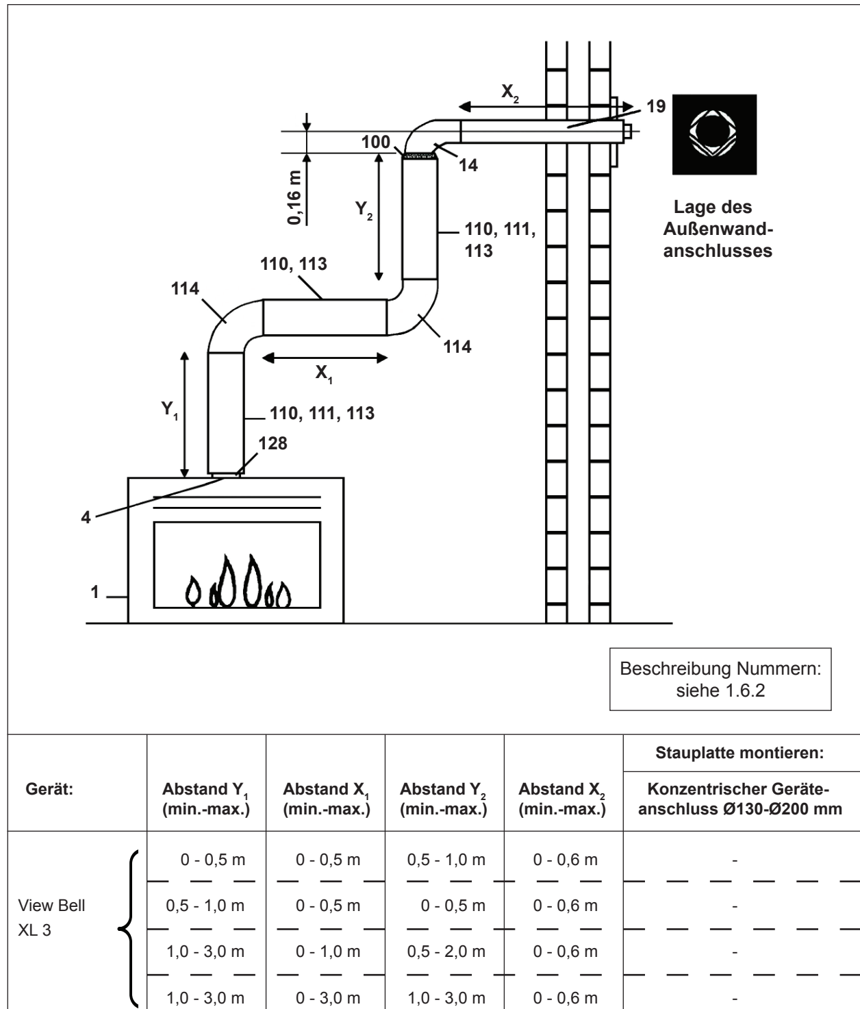
Abbildung 14: Horizontaler Außenwandanschluß
