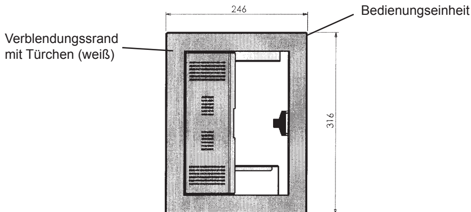
Abbildung 19: Bedienungseinheit
