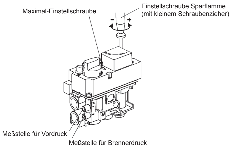
Abbildung 1: Gasregelblock Fernbedienung (Gerät mit Bedienungseinheit)
