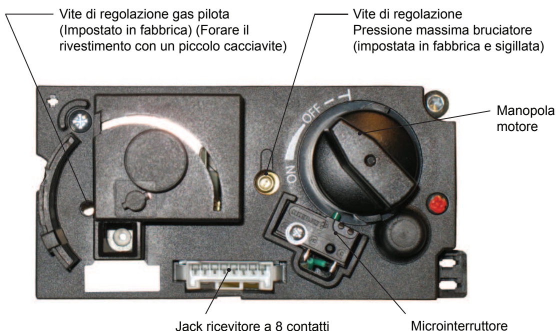
Figura 4: Blocco di regolazione gas
