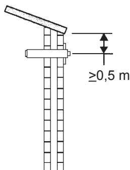
Abbildung 3: Abzug im Giebel
