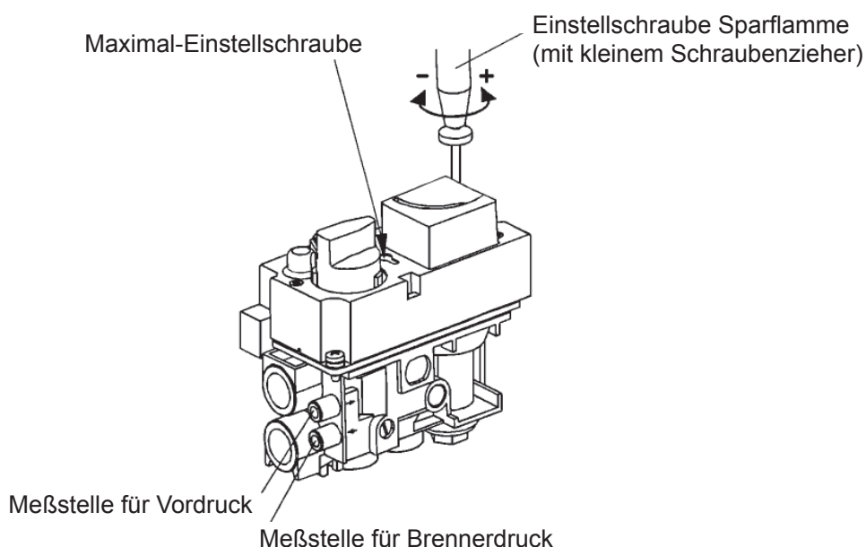
Abbildung 1: Gasregelblock Fernbedienung (Gerät mit Bedienungseinheit)
