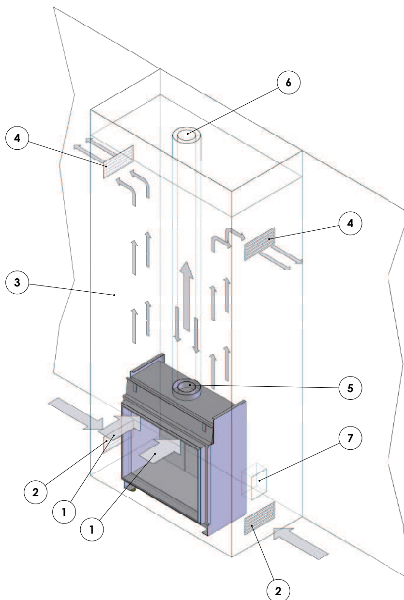
Figura 17: Apparecchio installata in canna fumaria ventilata Scarico verticale del gas bruciato / aria di combustione aspirata dal tetto. Montato senza kit di convezione
