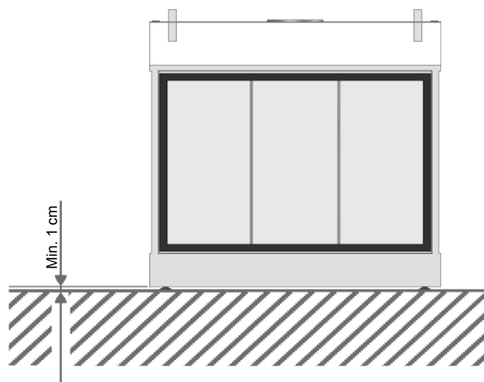
Figuur 15: Minimaal 1 cm ruimte tussen onderzijde toestel en vloer
