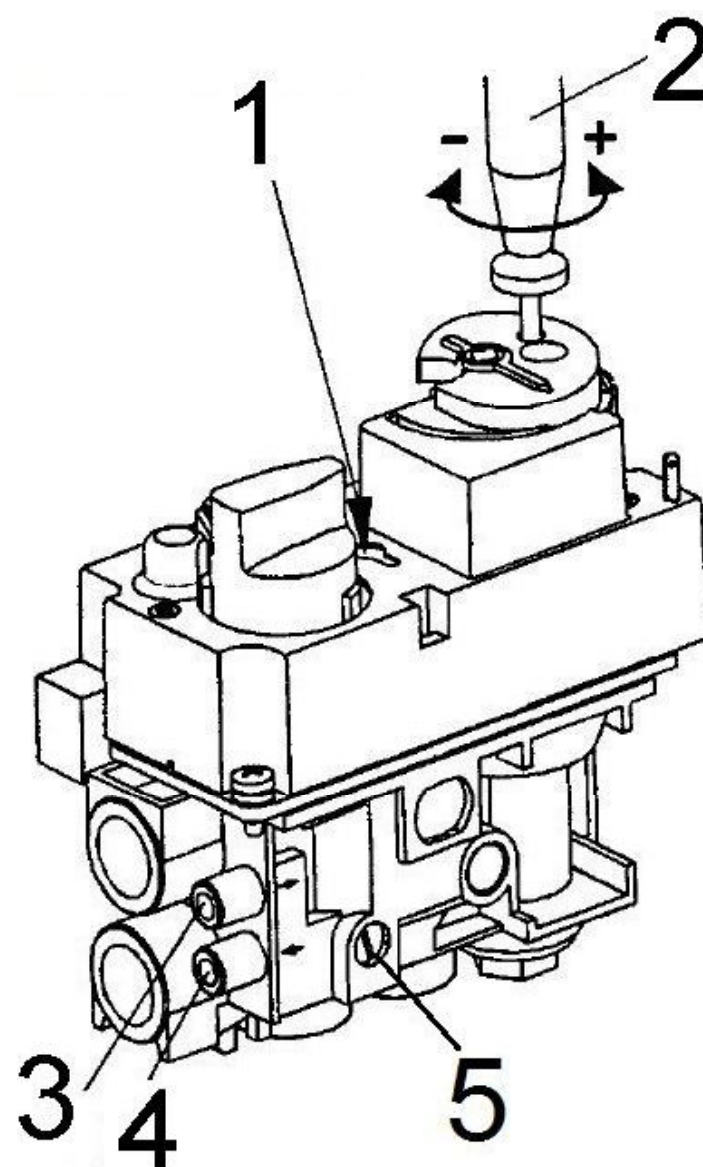
Abbildung 1: Gasregelblock
