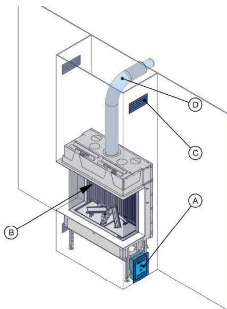
Abbildung 1: Typische Installation eines Gaskamins ohne Konvektionsmantel
