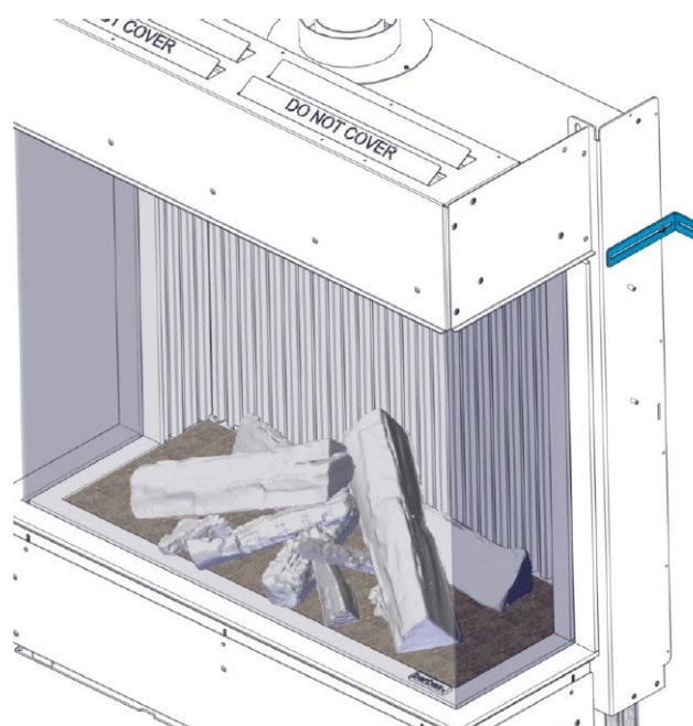
Abbildung 6: Befestigung an der Rückwand
