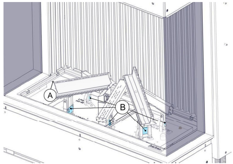
Abbildung 9: Positionen der Lufteinlass- und Primärlufteinlassöffnungen
