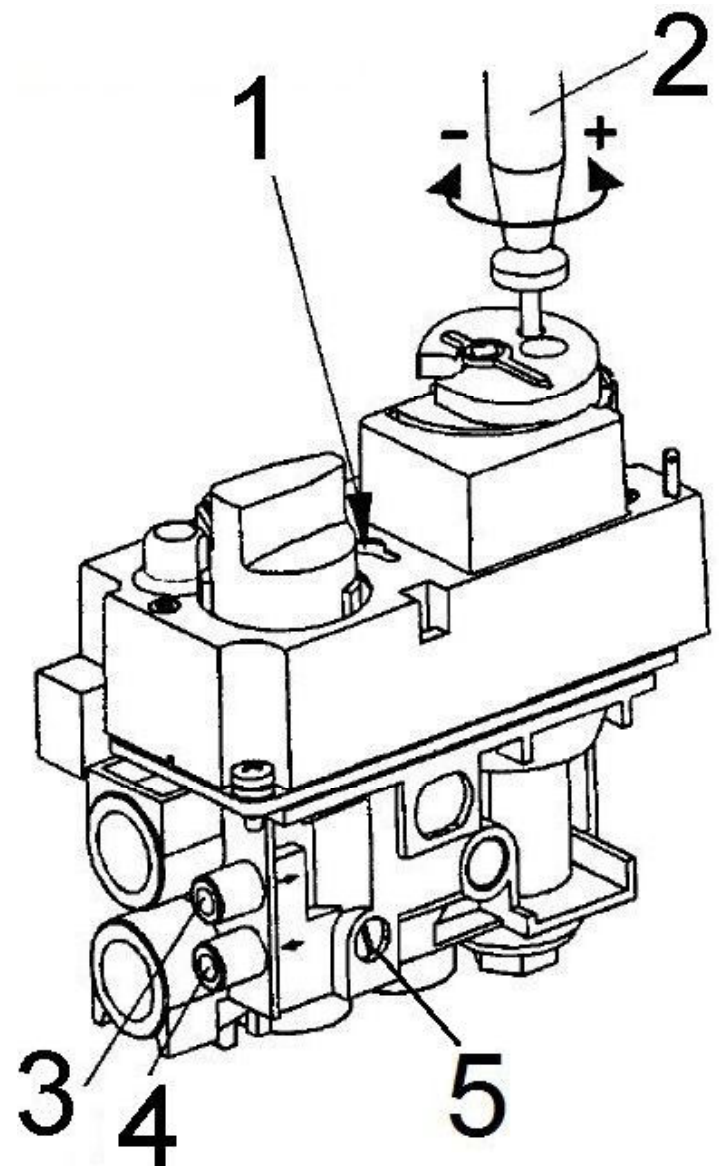
Abbildung 8: Gasregelblock
