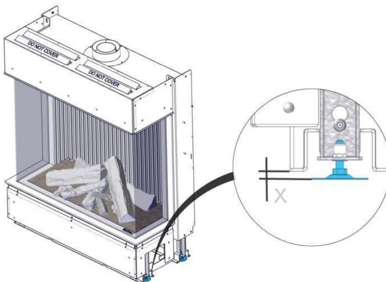
Abbildung 4: Ausrichtung mittels Stellfüßen
