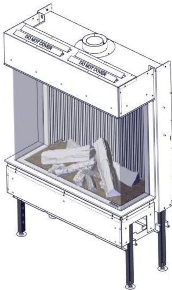
Abbildung 5: Ausrichtung mittels höhenverstellbarer Füße
