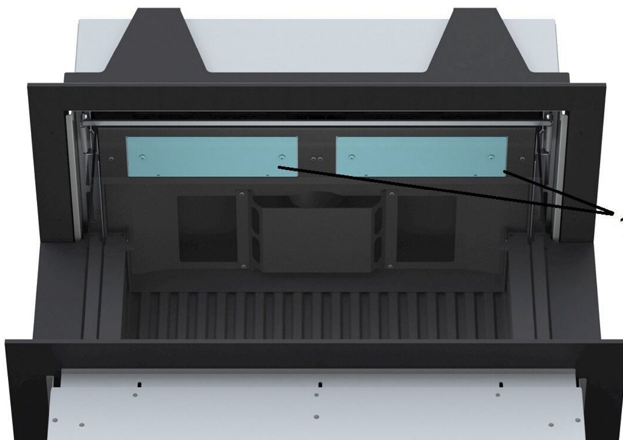
Abbildung 7: Überdruckklappen (1)
