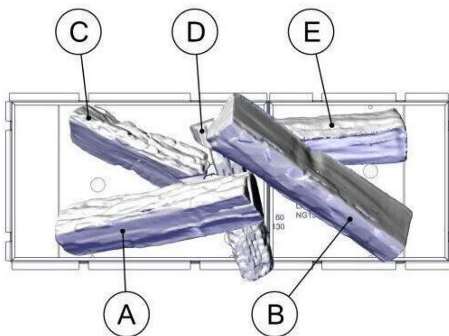
Abbildung 10: Positionen der Holzimitate und Brennerleisten
