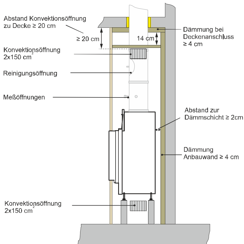
Aufbau vor oder neben einer sonstigen Wand/Decke:
