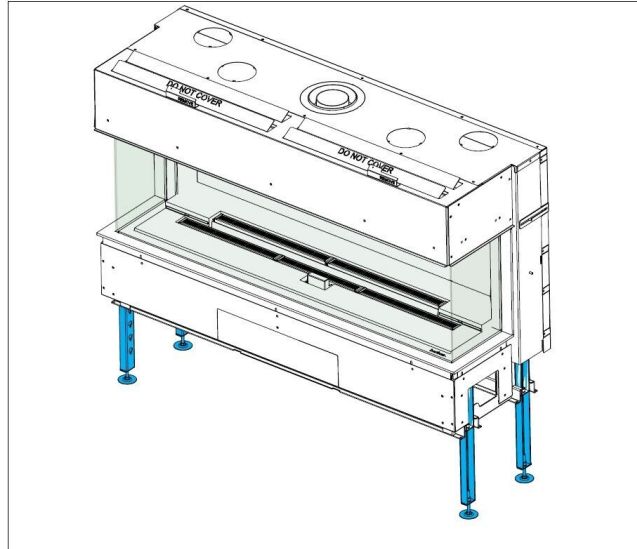
Abb. 9: Ausrichtung mittels höhenverstellbarer Füße
