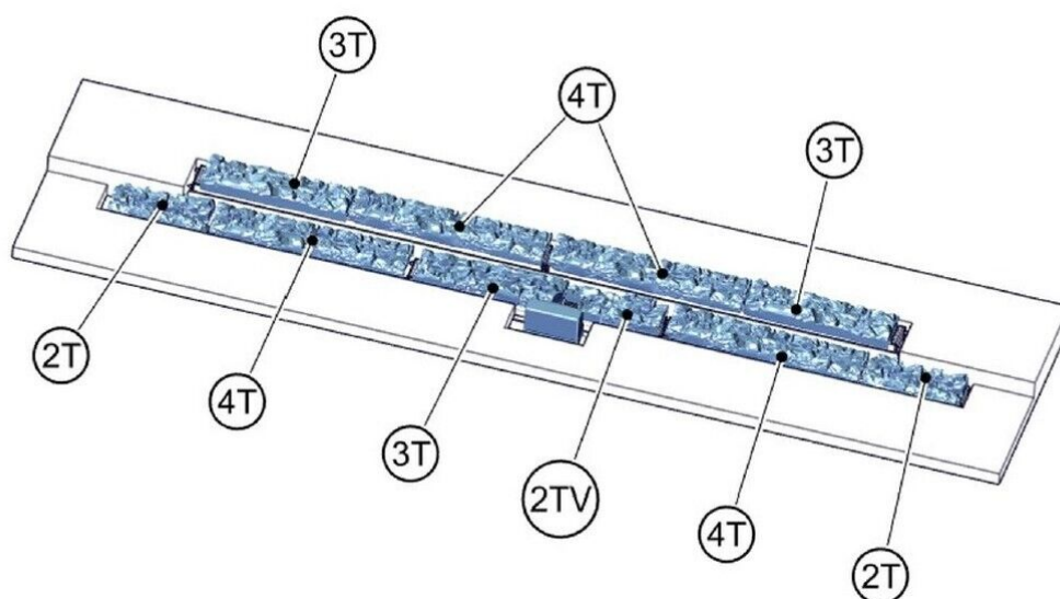
Abb. 4: Position der Glutroste und Glutimitat, gleichmässig um die Glutroste verteilt
