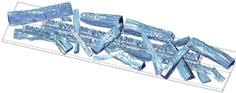
Abb. 13: Positionen der Holzimitate und Brennerleisten
