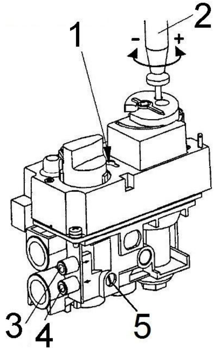
Abbildung 1: Gasregelblock
