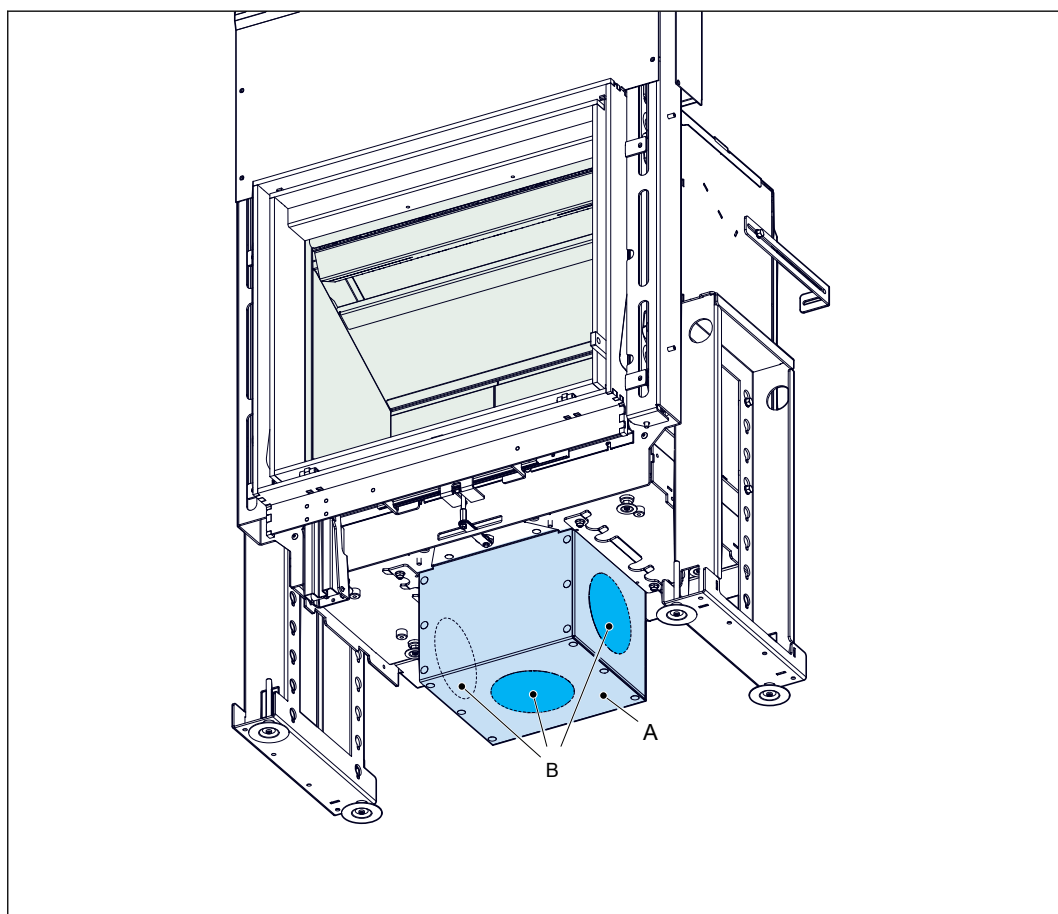
A Boîtier d'entrée d'air de combustion B Entrée d'air de combustion
