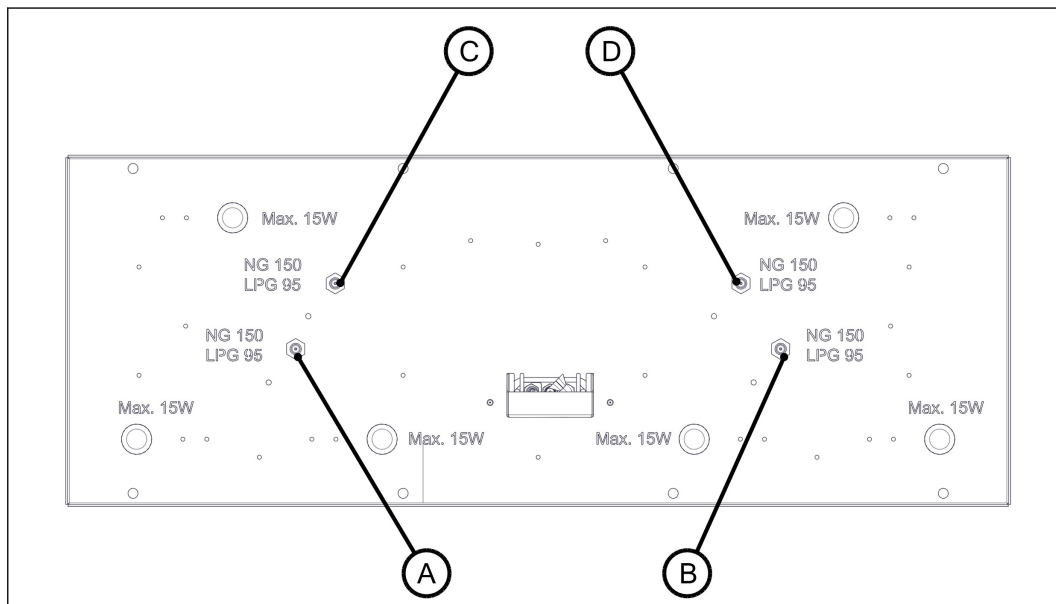
Figure 40. Position des entrées d'air primaires et des injecteurs de gaz
