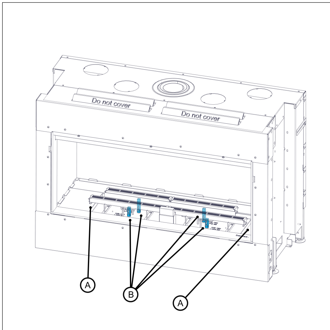
Figure 35. Positionnement des ouvertures d'entrée d'air primaire et d'admission d'air
