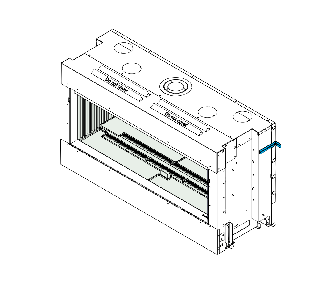
Figure 28. Fixation sur paroi arrière
