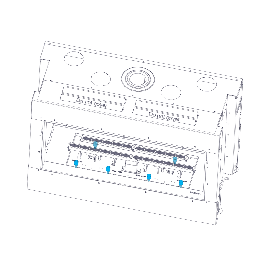
Figure 38. Positionnement d'ampoules d'éclairage d'ambiance
