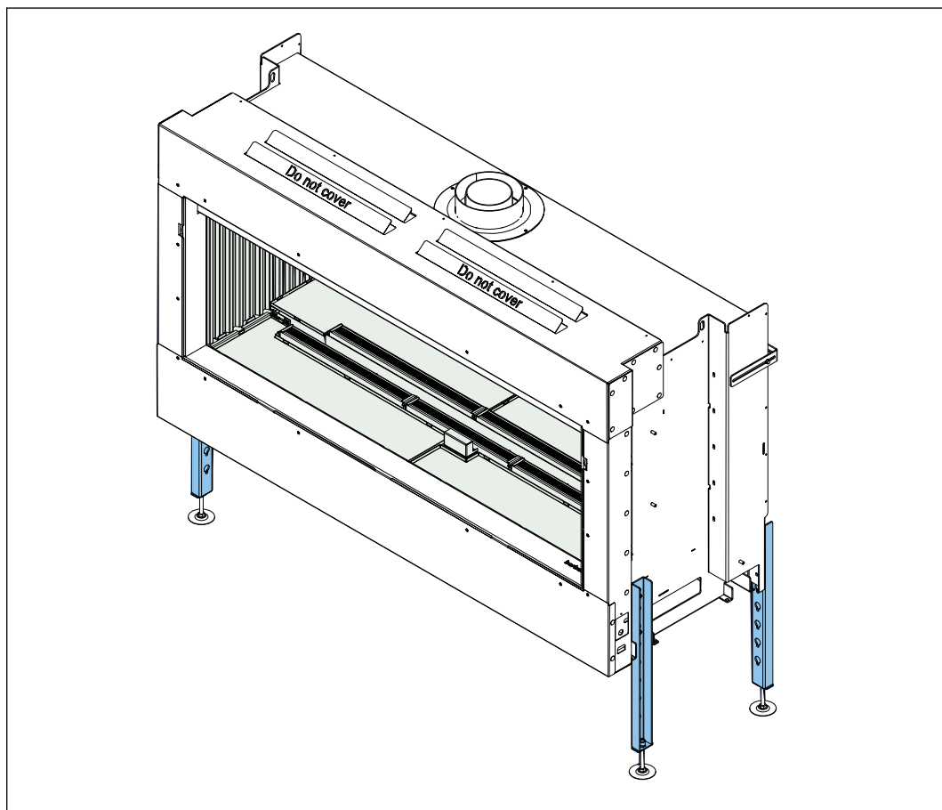
Figure 27. Alignement avec pattes réglables en hauteur
