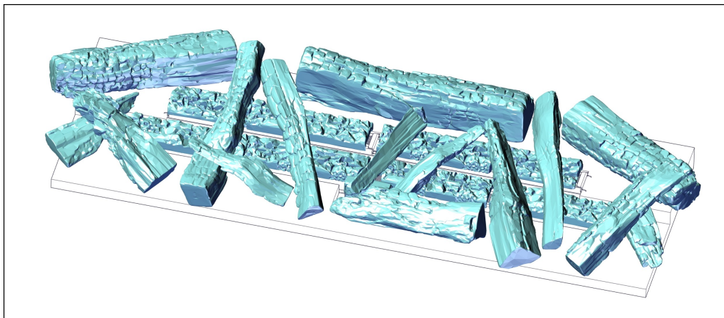
Figure 37. Positionnement des bûches de bois céramiques et des brûleurs
