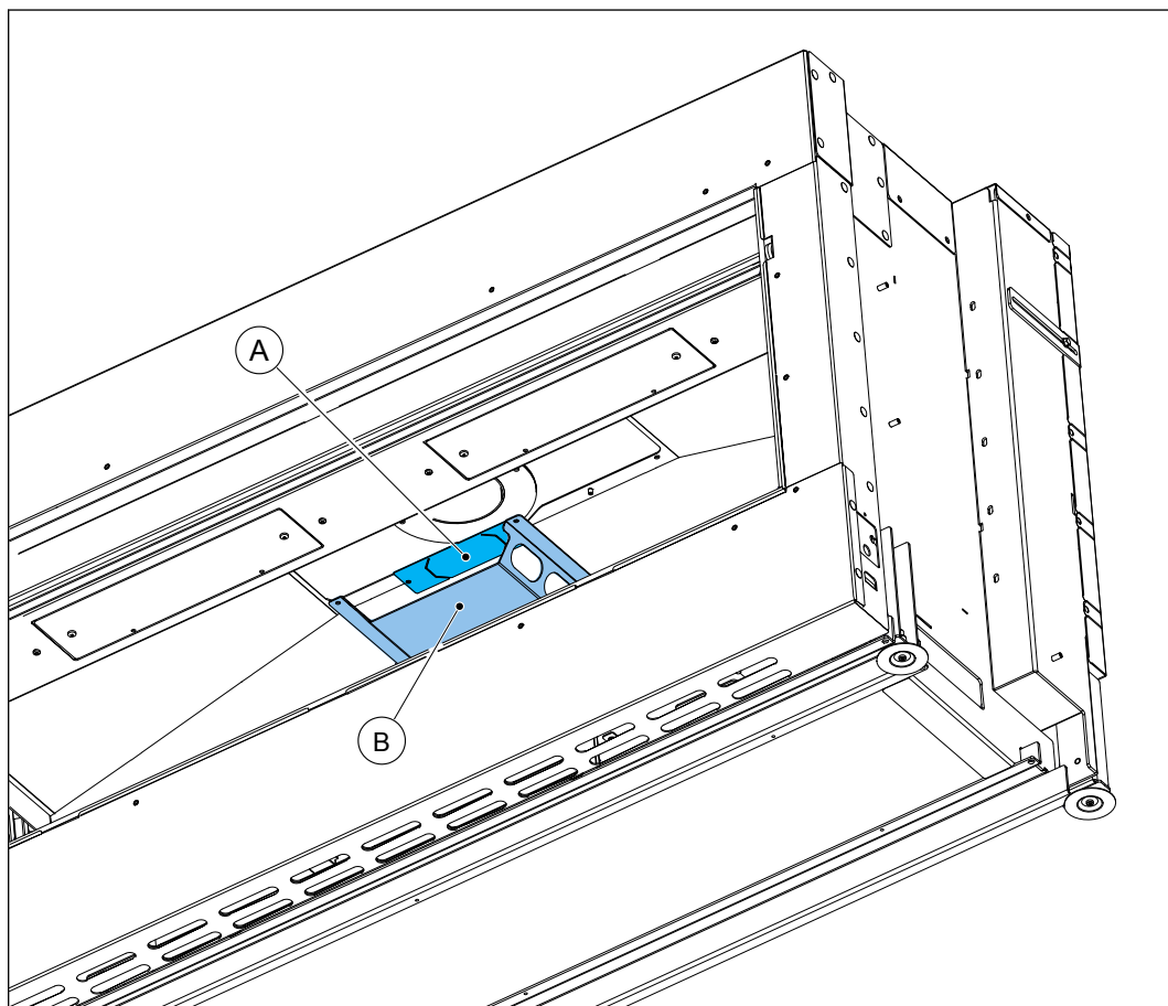
Figure 32. Déflecteur et plaque de restriction
