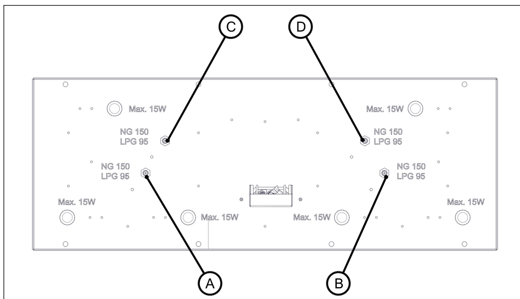
Figure 39. Position des entrées d'air primaires et des injecteurs de gaz
