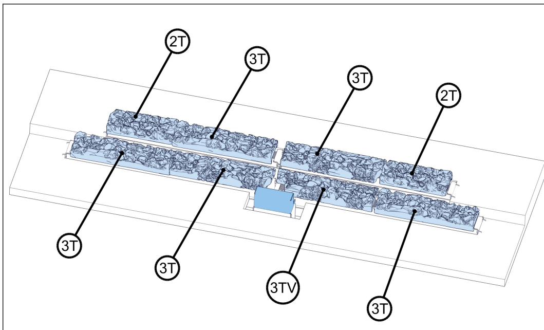
Position des grilles de braise et du verre à feu ; distribution uniforme autour des grilles de braise
