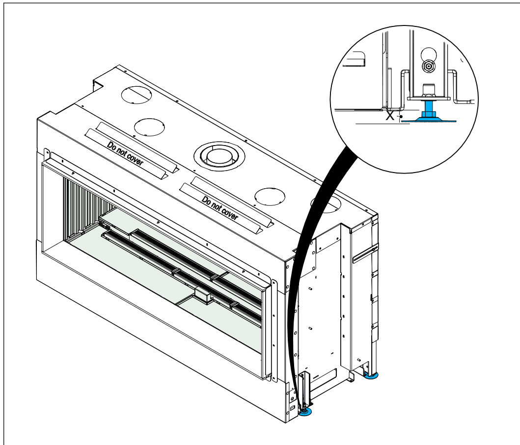
Figure 26. Alignement avec pieds réglables
