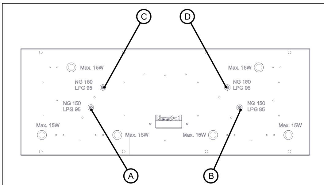
Figura 39. Posizioni degli ingressi dell'aria principali e degli iniettori di gas
