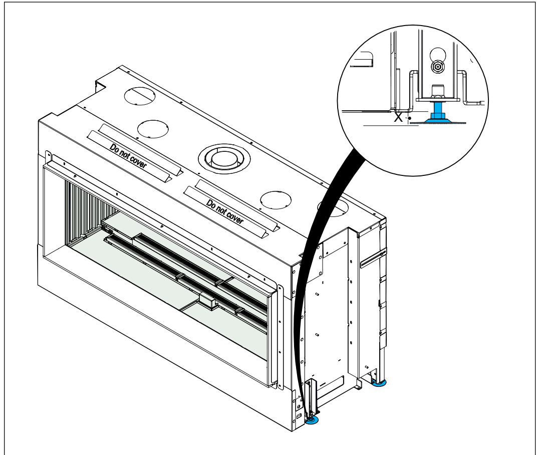
Figuur 26. Uitlijnen met behulp van stelvoeten
