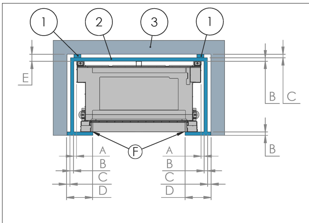
Figuur 14. Afstanden tot niet-brandbare wand – Bovenaanzicht
