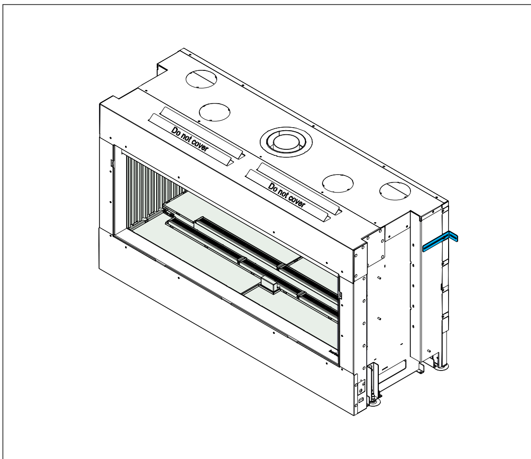
Figuur 28. Bevestiging aan de achterwand
