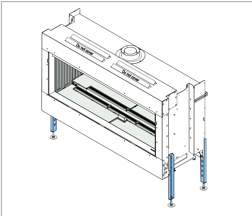
Figuur 27. Uitlijnen met behulp van de stelvoeten
