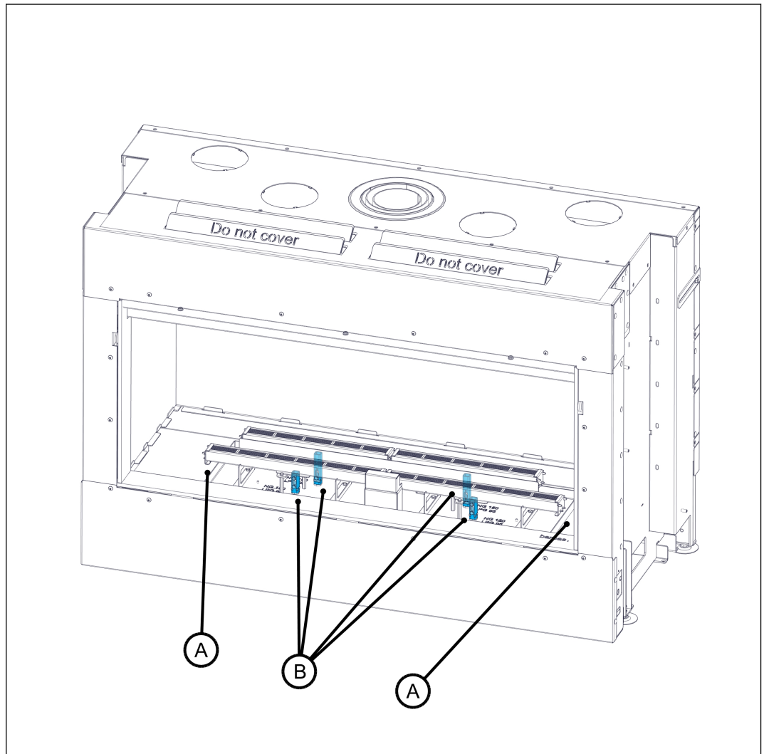
Figuur 35. Positie van luchtinlaat- en primaire luchtinlaatopeningen
