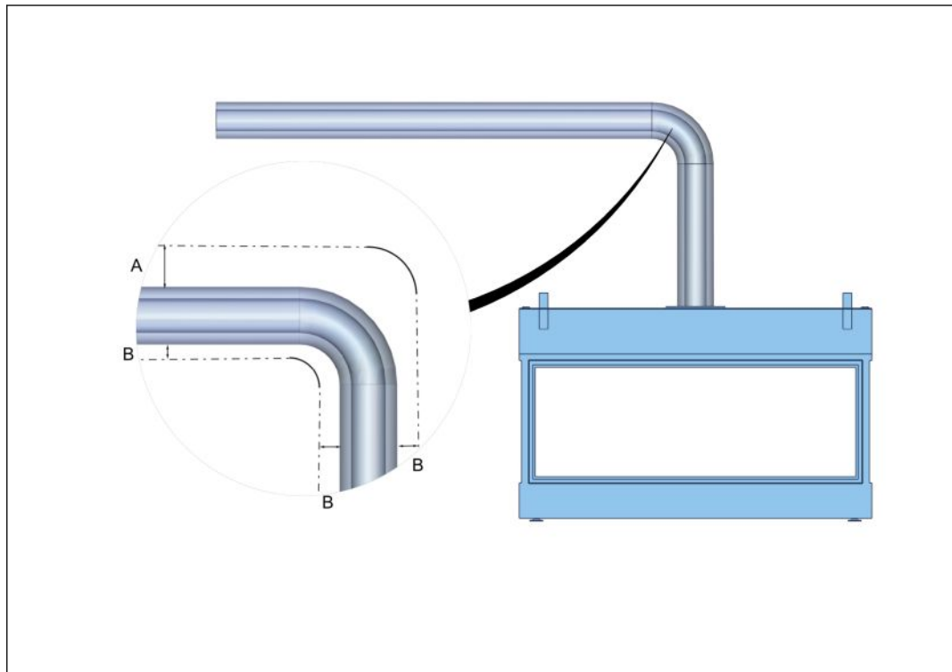
Figuur 20. Vrije ruimtes concentrisch rookkanaal
