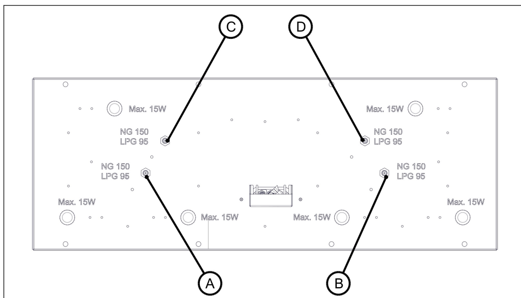
Figuur 39. Positie van primaire luchtinlaten en gasinjectoren
