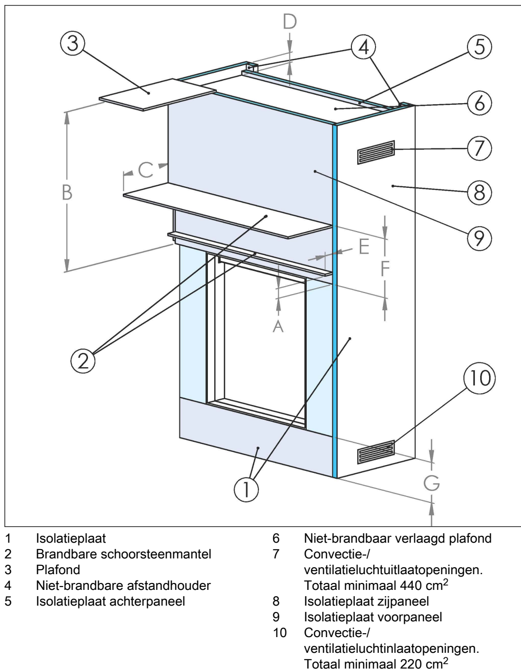
Figuur 17. Vrije ruimtes voor de schoorsteenmantel
