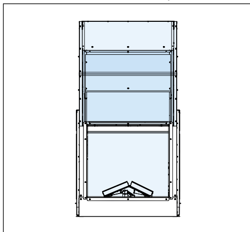
Abbildung 9. Serviceposition Kaminschirm
