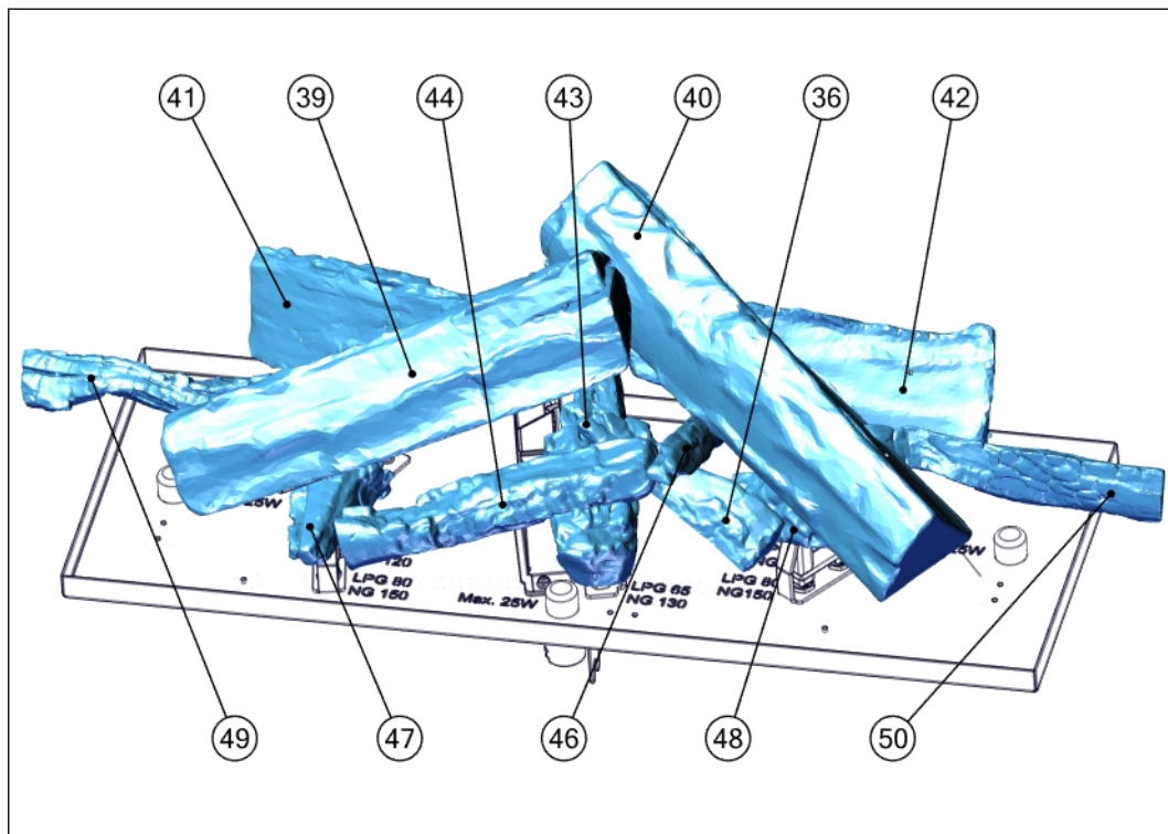
Figura 4. Vista general del kit de troncos cerámicos
