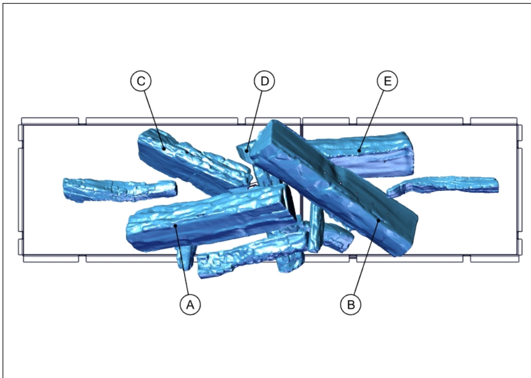
Figura 45. Posición de los troncos de madera cerámica y los quemadores
