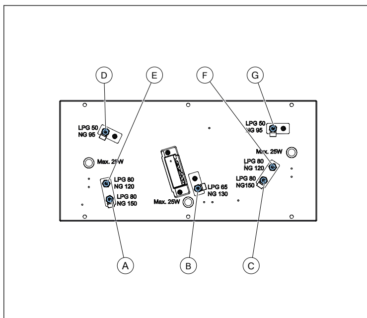
Figuur 48. Positie van primaire luchtinlaten en gasinjectoren
