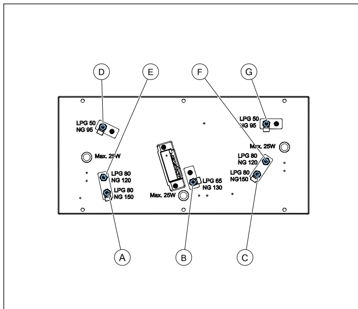
Figure 48. Position des entrées d'air primaires et des injecteurs de gaz
