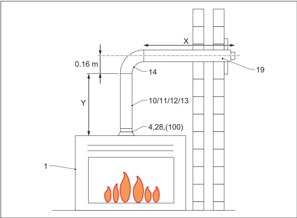
Collegamento della canna fumaria concentrica sull'apparecchio da Ø100-Ø150 mm o Ø130-Ø200 mm
