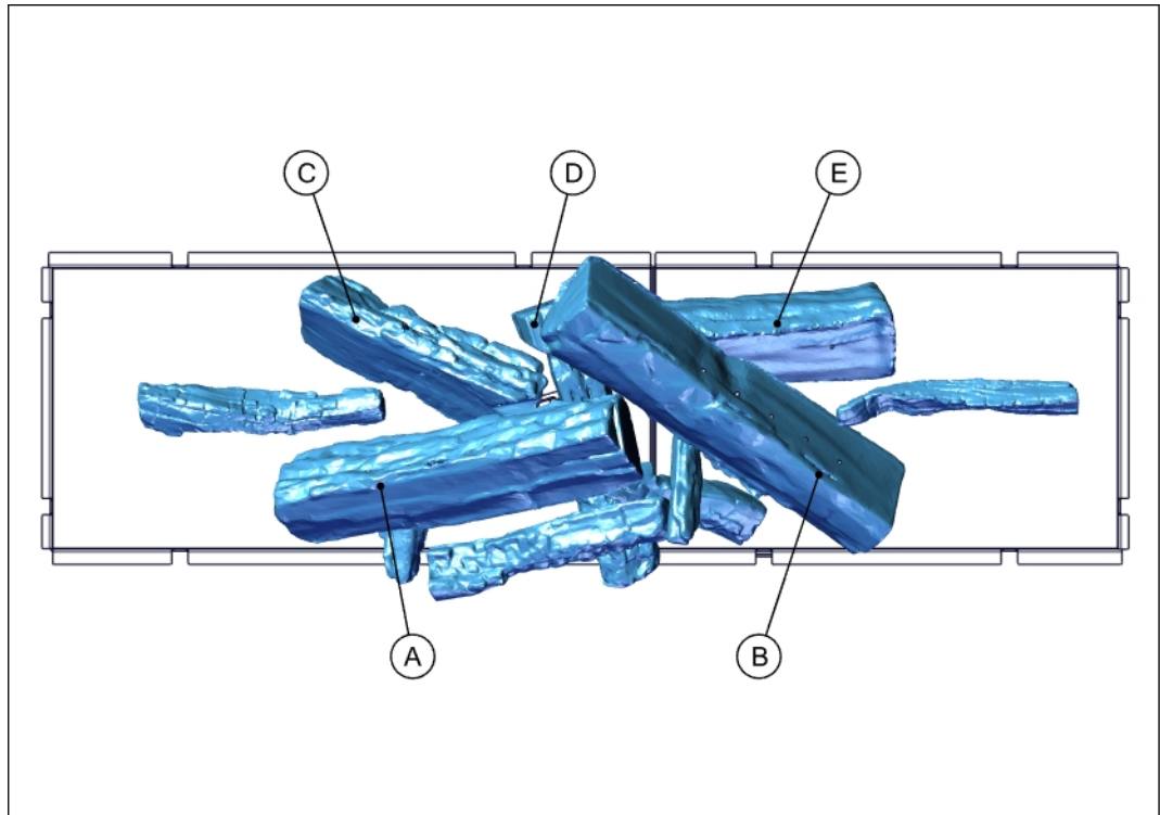
Figuur 45. Positie van keramische houtstammen en branders
