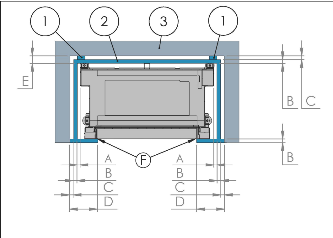
1 Espaceur inflammable 3 Paroi inflammable 2 Plaque d'isolation inflammable
