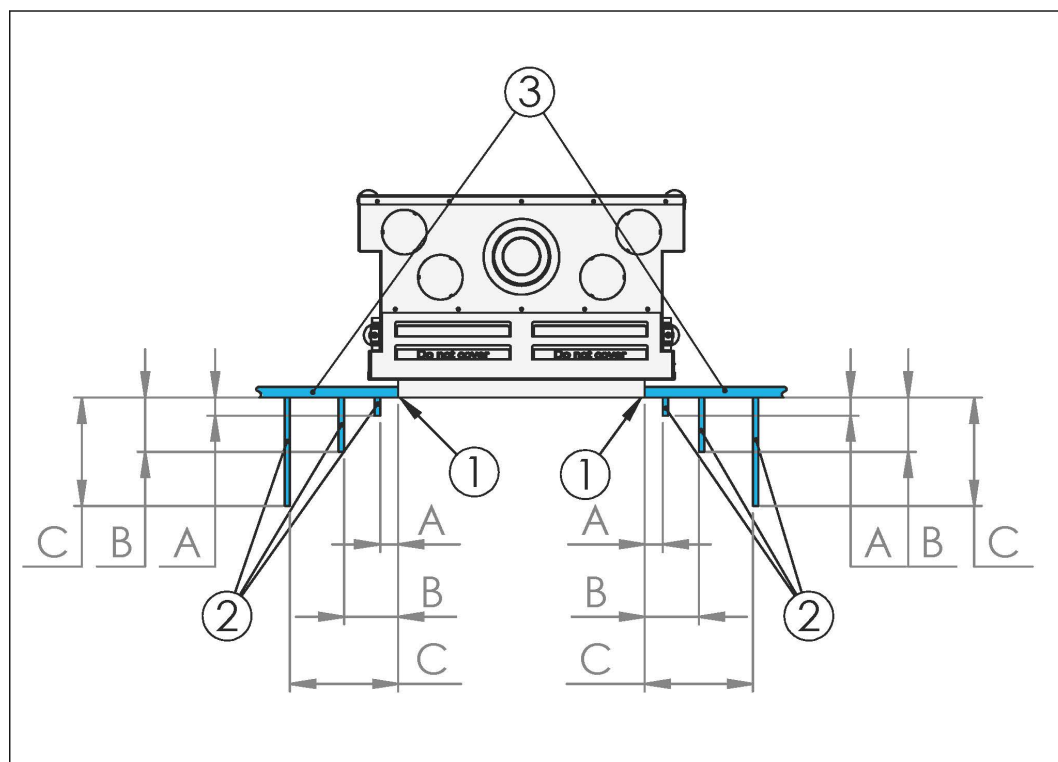
1 Côté de panneau de verre avant 3 Plaque d'isolation 2 Manteau inflammable
