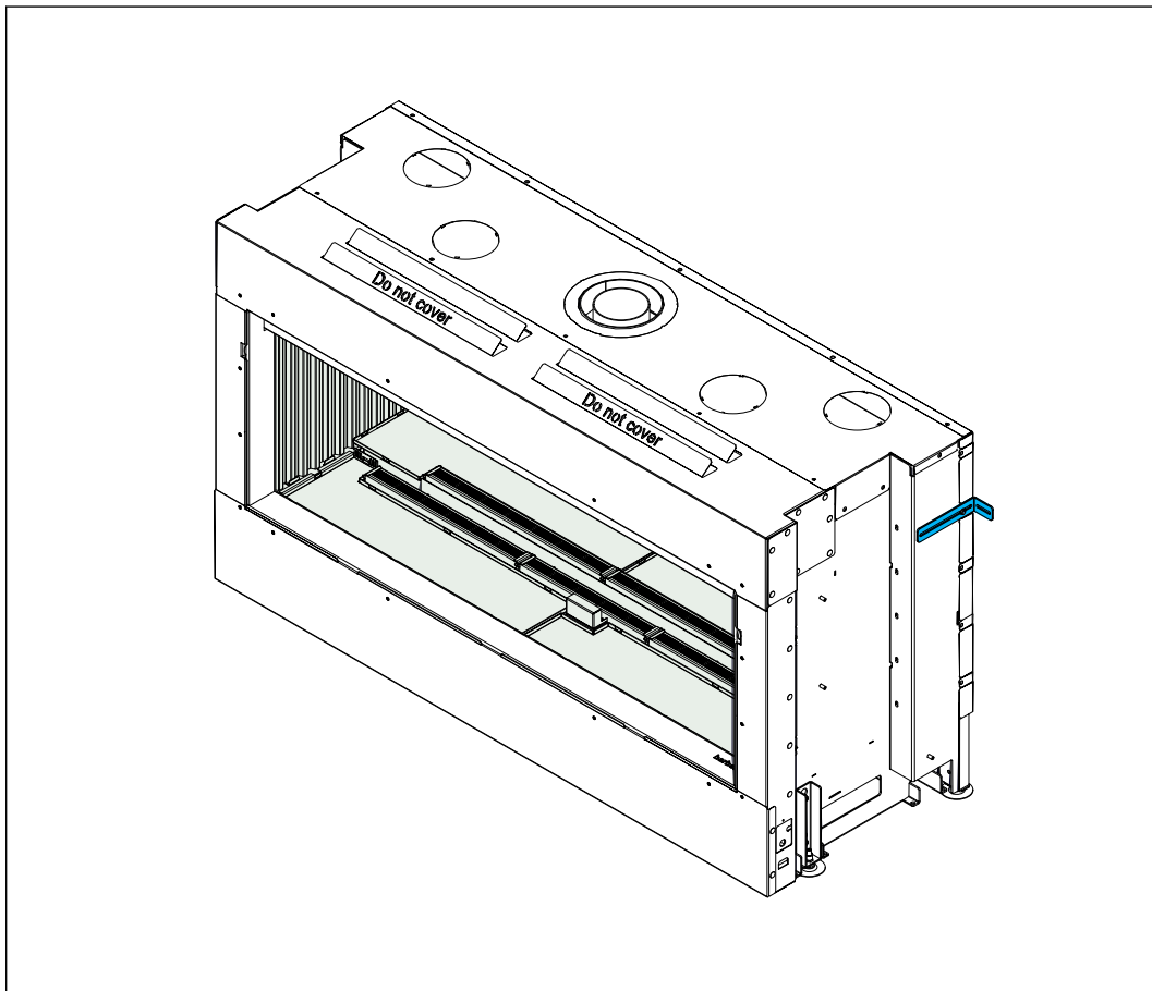
Figura 28. Fijación a la pared posterior
