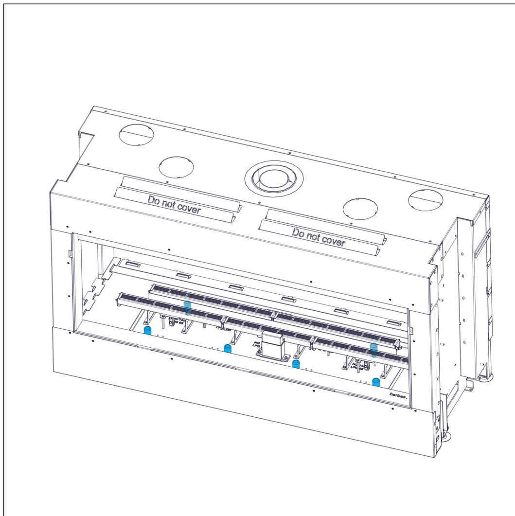
Figura 38. Posición de las bombillas de luz ambiental
