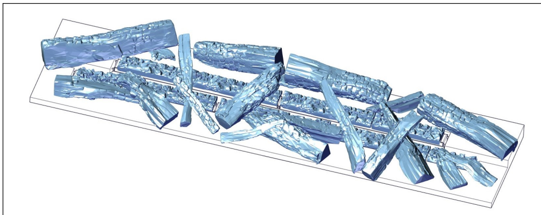
Figura 37. Posición de los troncos de madera cerámica y los quemadores
