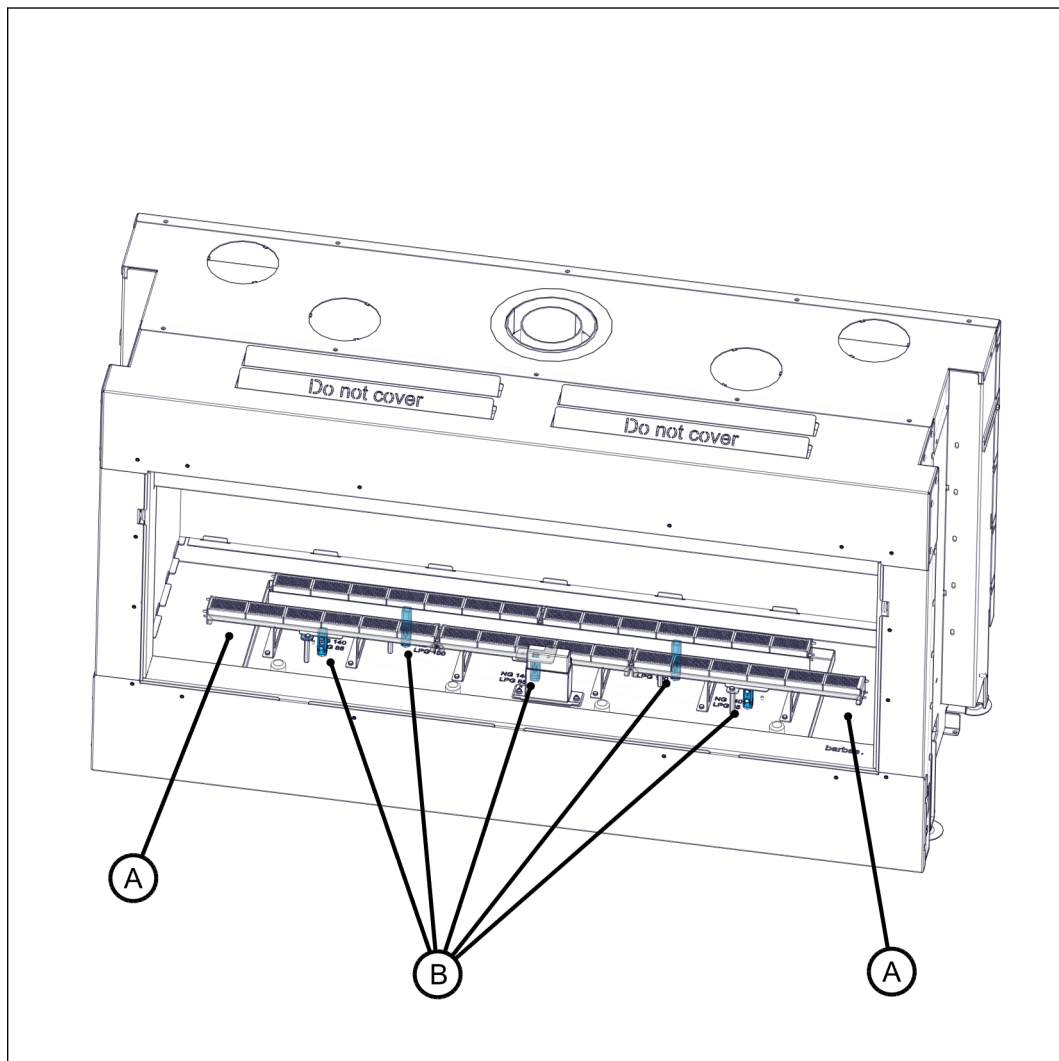
Figura 35. Posición de la entrada de aire y las aberturas de entrada de aire principales
