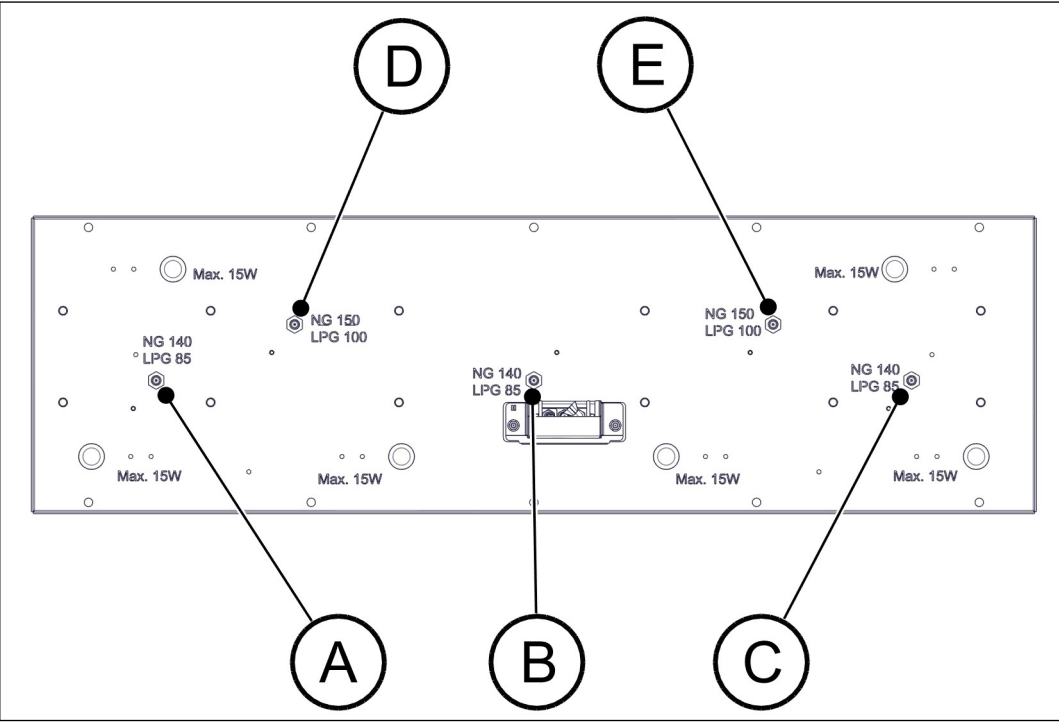
Figura 39. Posición de las entradas de aire principales y los inyectores de gas
