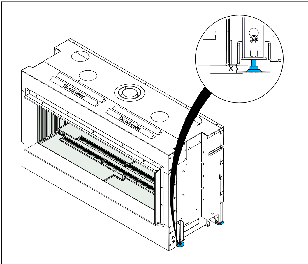
Figura 26. Alineación con los pies ajustables
