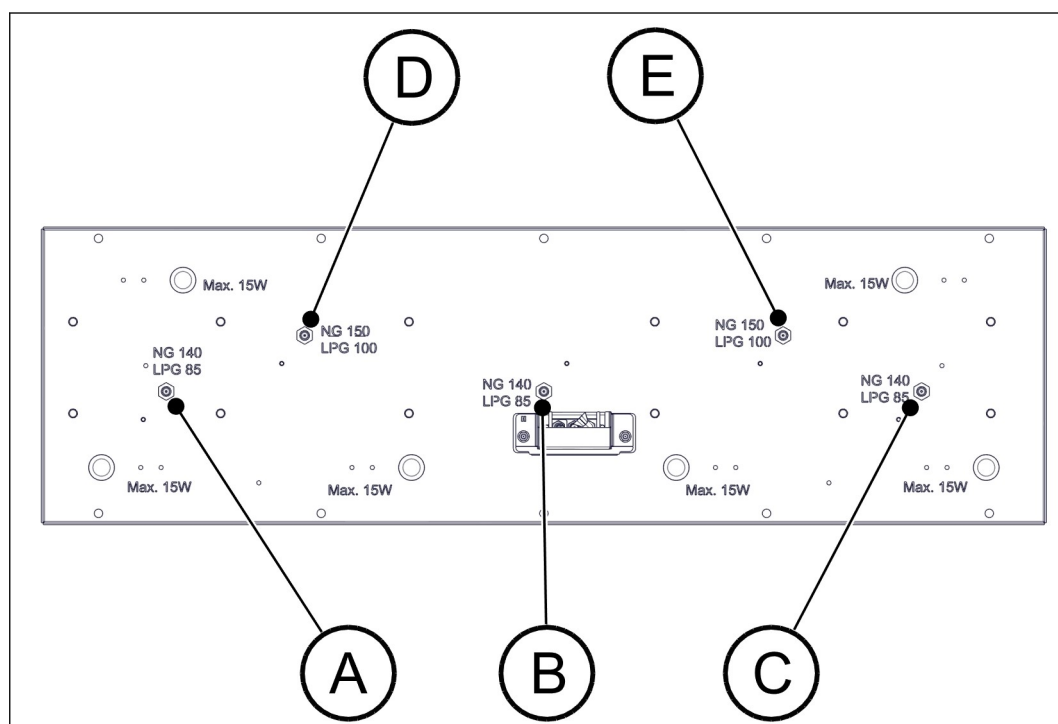
Figure 39. Position des entrées d'air primaires et des injecteurs de gaz
