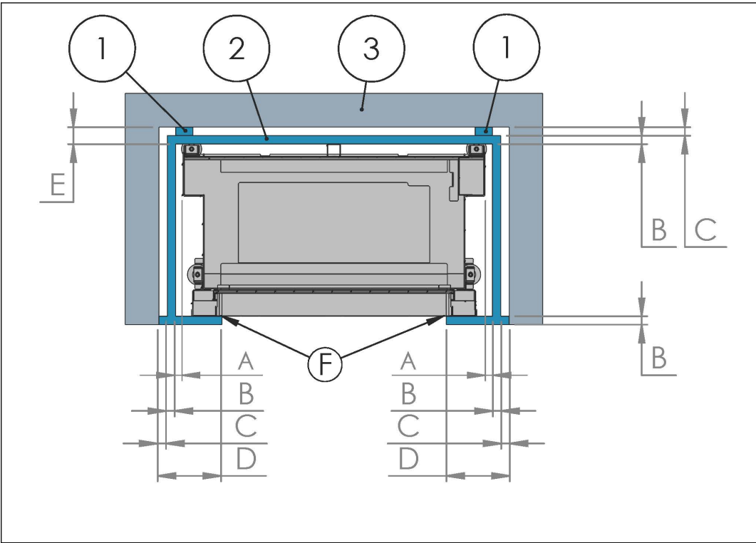
1 Espaceur inflammable 2 Plaque d'isolation inflammable 3 Paroi inflammable
