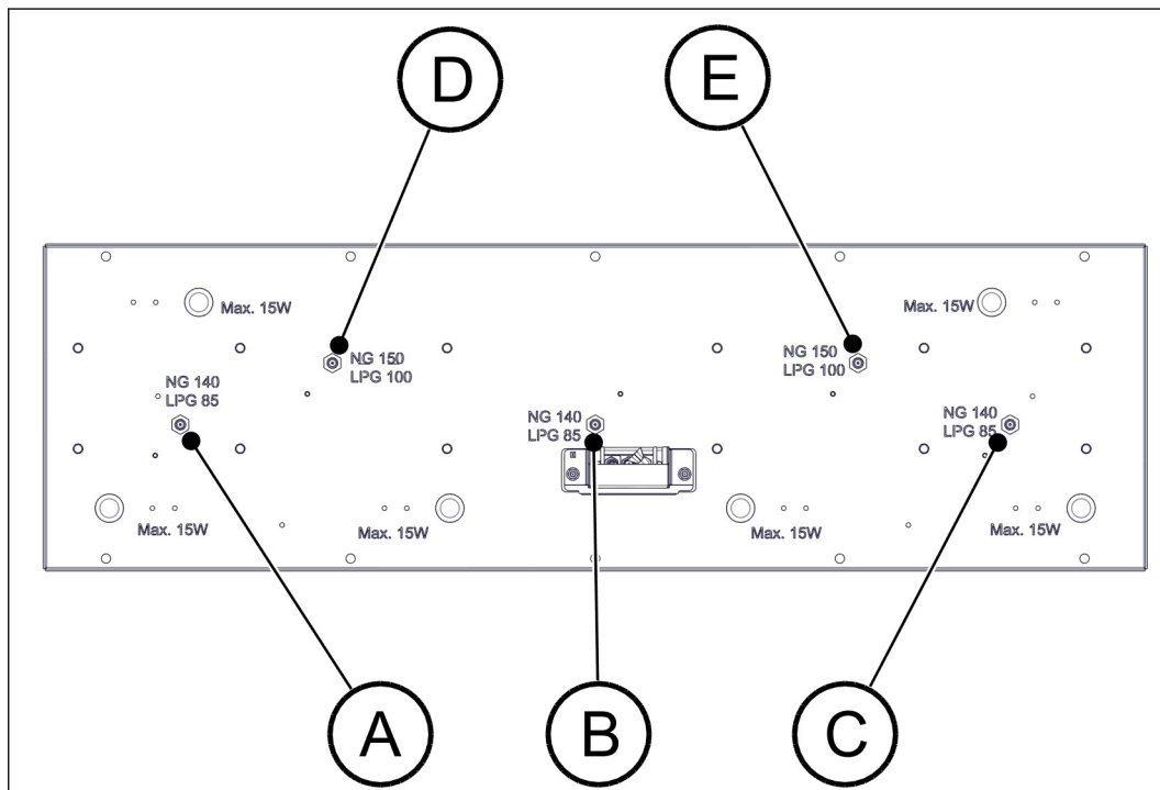
Figure 40. Position des entrées d'air primaires et des injecteurs de gaz
