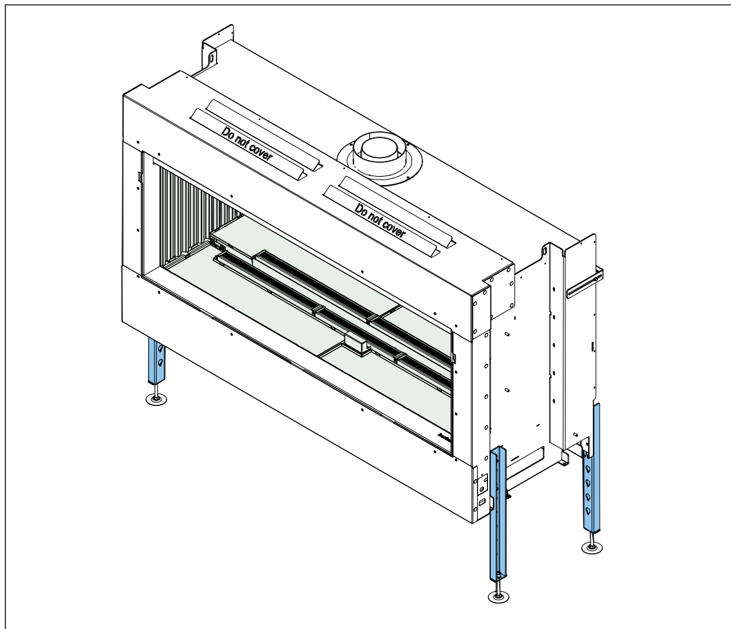
Figura 27. Allineare con le gambe ad altezza regolabile
