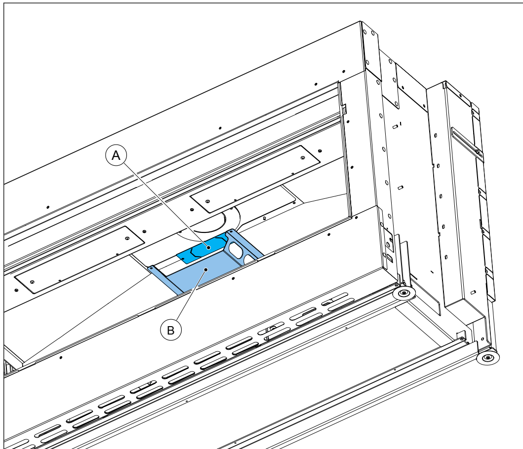
Figura 32. Piastra di restrizione e pannello deflettore
