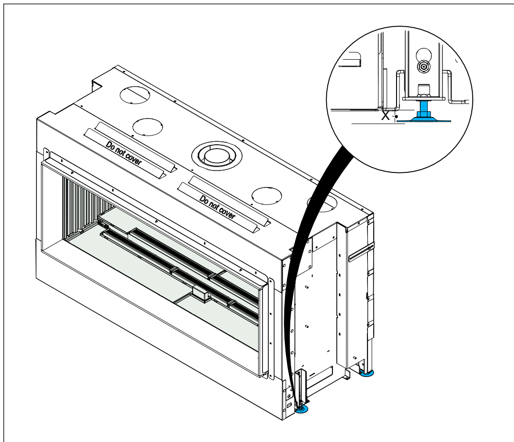
Figura 26. Allineamento con i piedini regolabili
