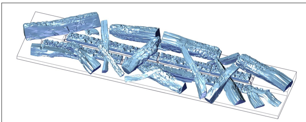
Figura 4. Panoramica del set di tronchetti in fibra ceramica
