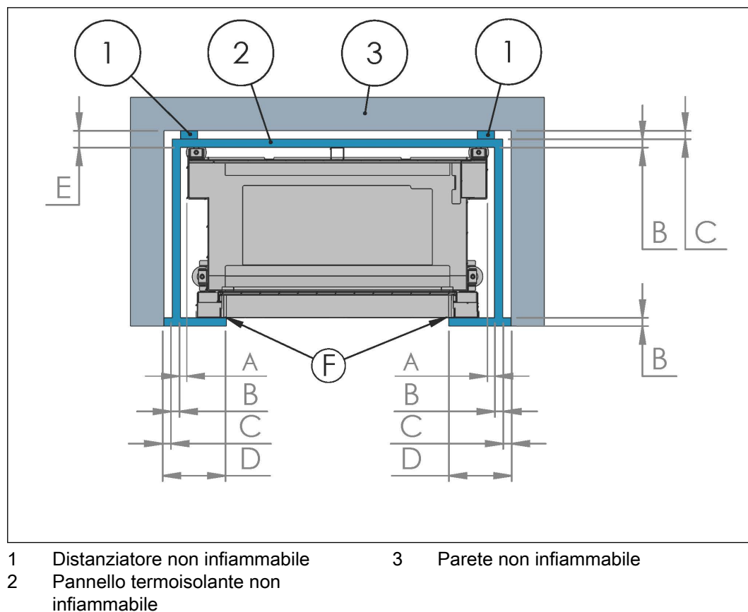
Figura 14. Distanze da pareti non infiammabili - Vista superiore
