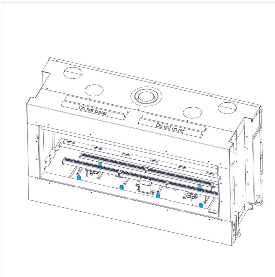
Figura 38. Posizione delle lampade per l'illuminazione ambiente
