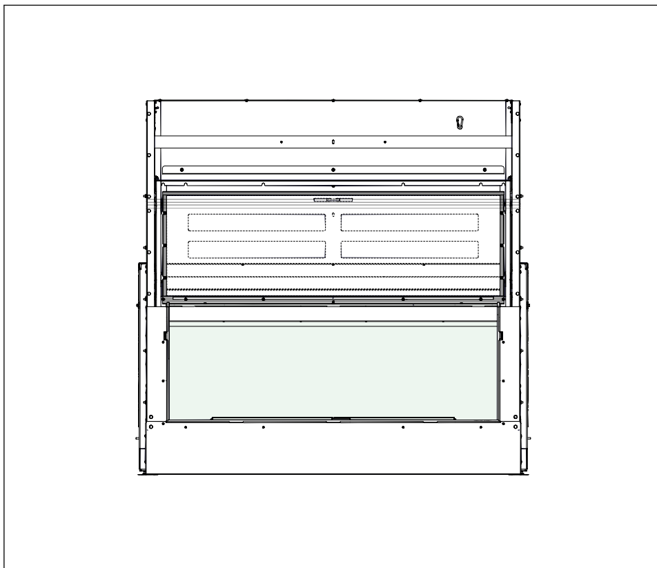
Figura 36. Schermo del camino nella posizione di servizio
