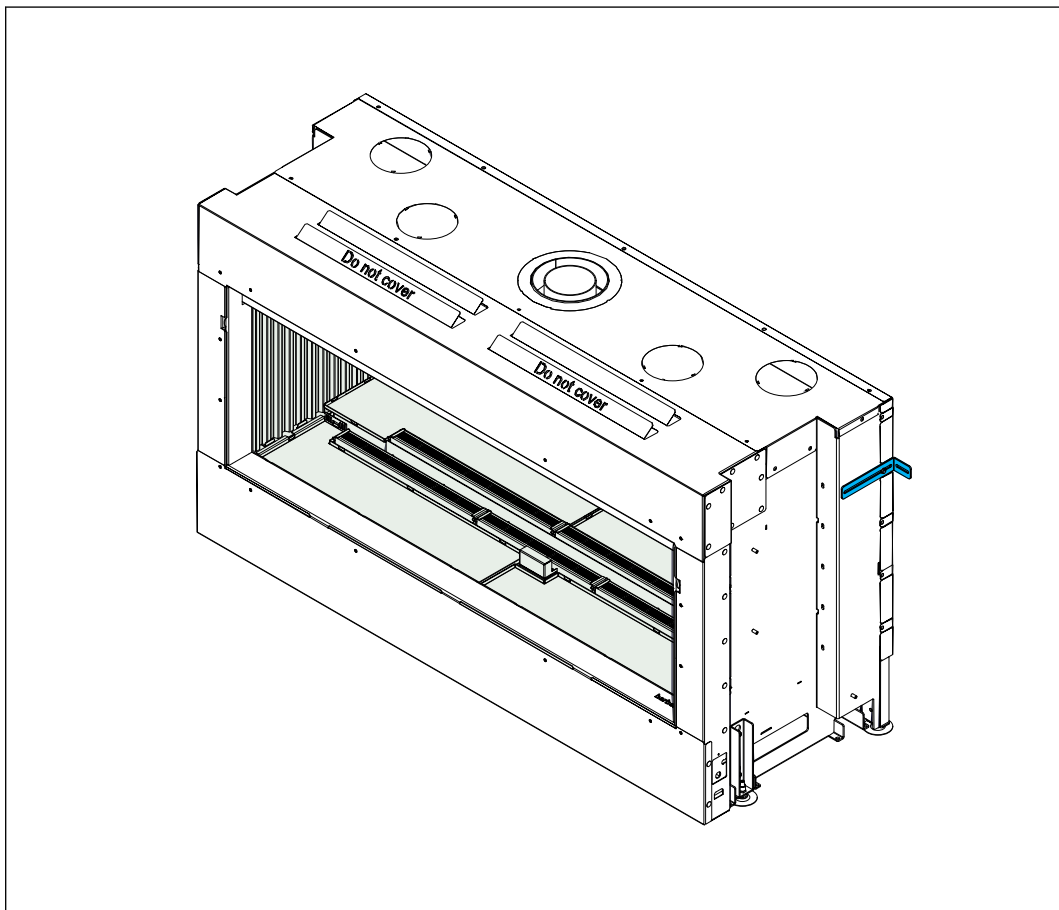
Figura 28. Fissaggio alla parete posteriore
