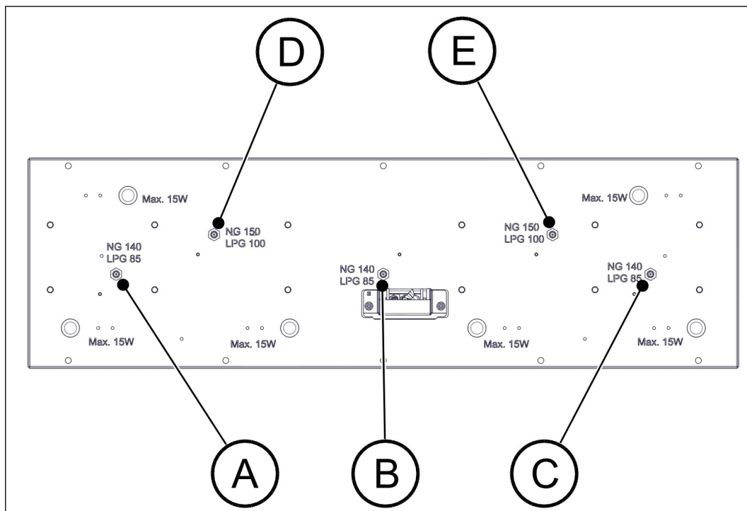
Figura 39. Posizioni degli ingressi dell'aria principali e degli iniettori di gas
