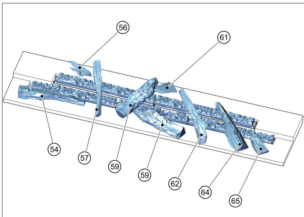
Positie van de houtstammen - Stap 1
