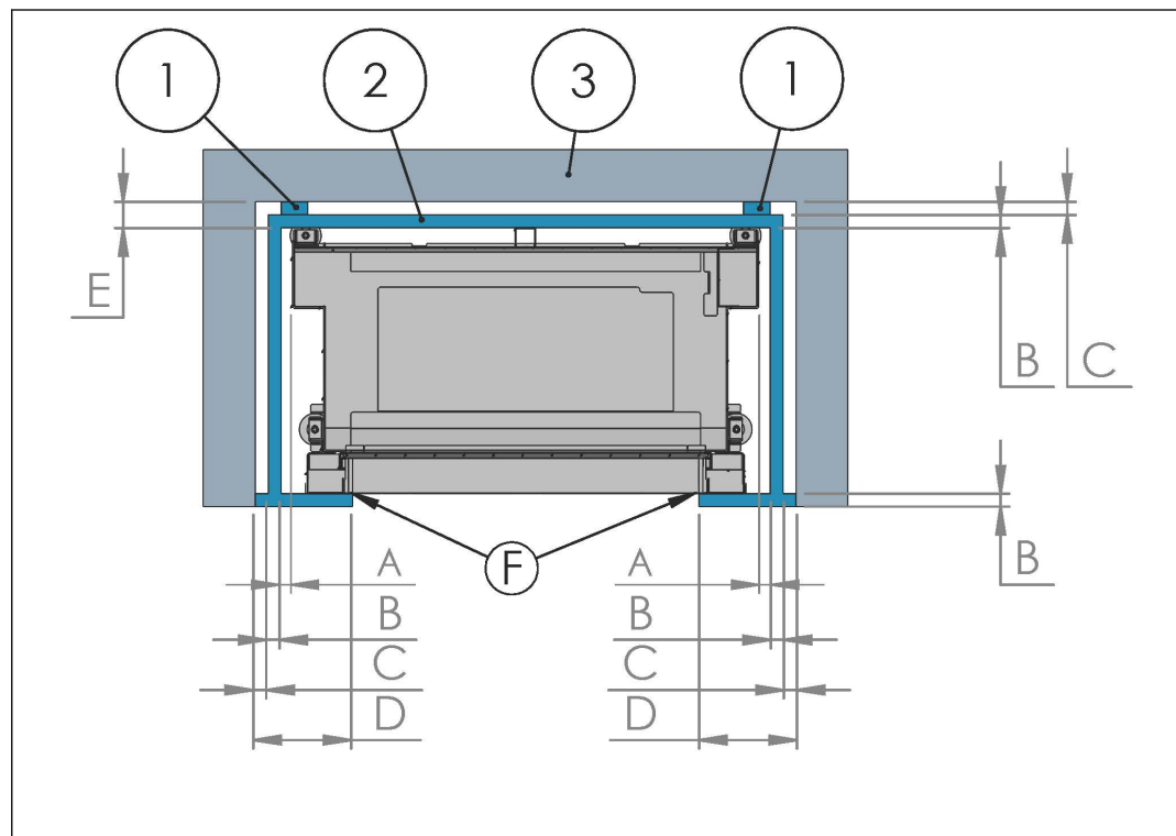
Abbildung 12. Abstände zur brennbaren Wand – Draufsicht
