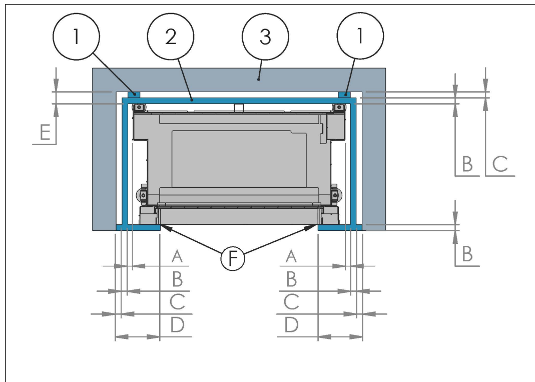
1 Espaceur ininflammable 3 Paroi inflammable 2 Plaque d'isolation ininflammable
