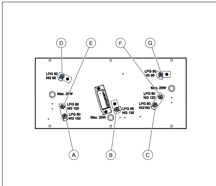
Abbildung 48. Positionen der Primärlufteinlässe und Gasinjektoren
