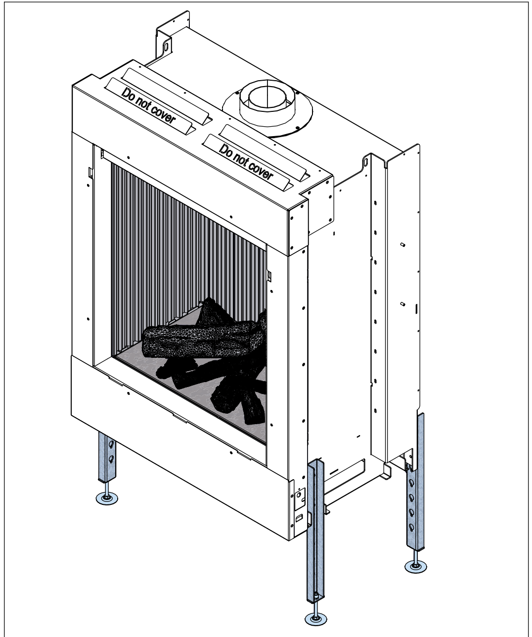
Abbildung 27. Ausrichtung mithilfe höhenverstellbarer Füße
