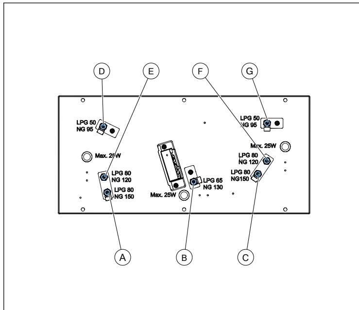
Abbildung 46. Positionen der Primärlufteinlässe und Gasinjektoren
