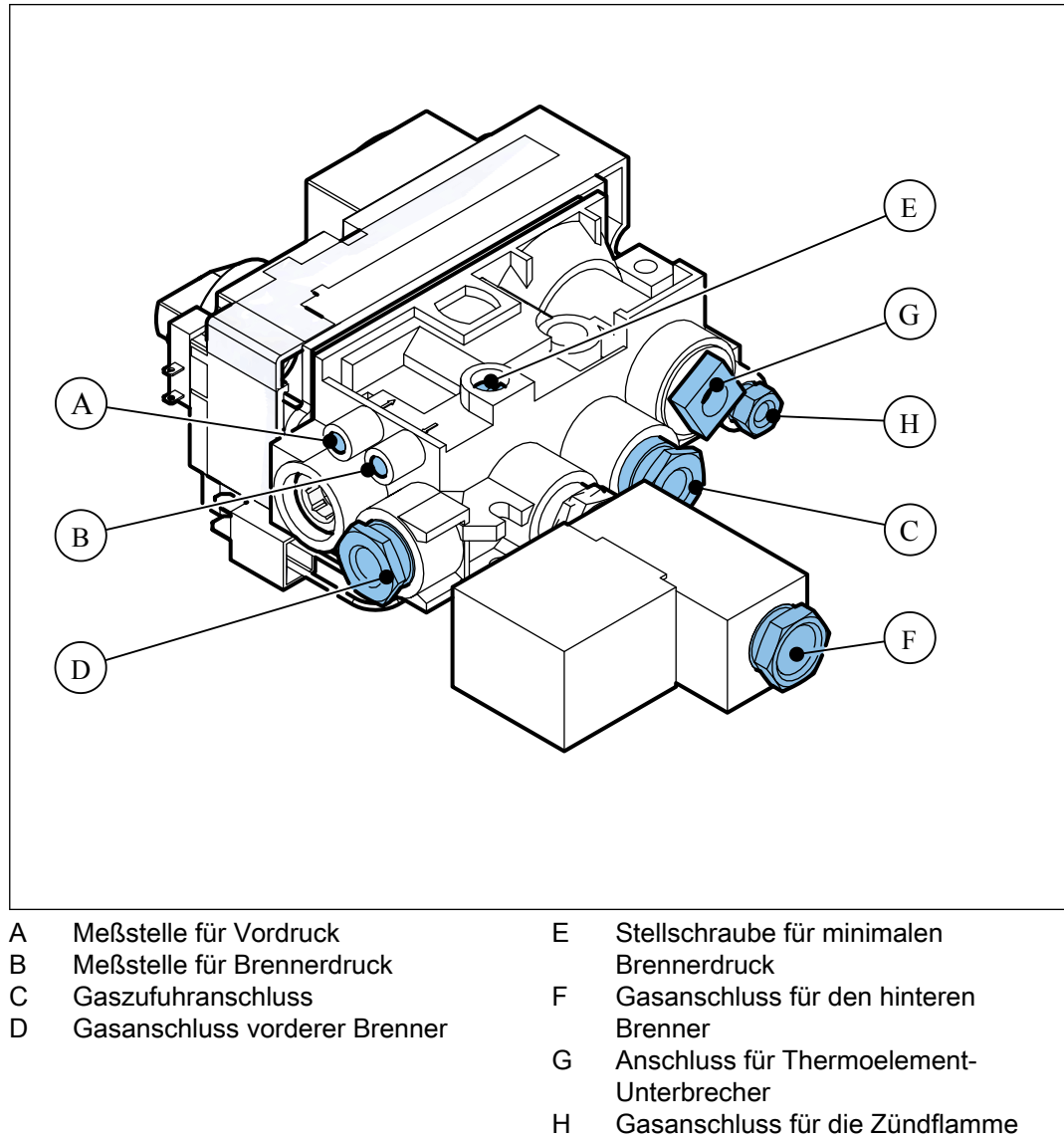
Abbildung 5. Gasreglerblock (hinten)
