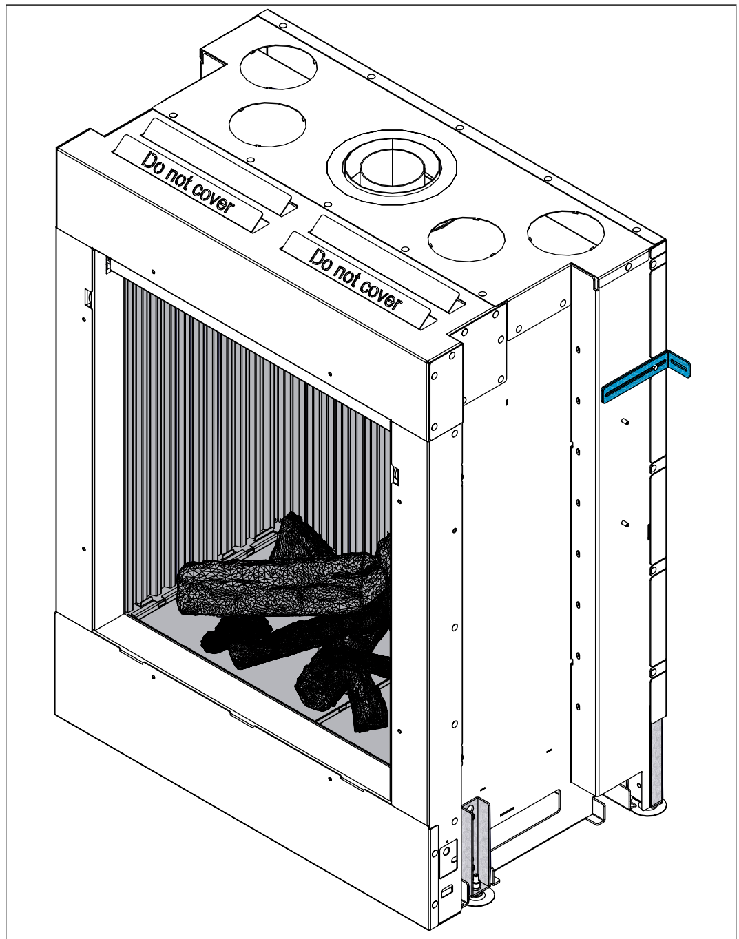
Abbildung 28. Befestigung an der Rückwand
