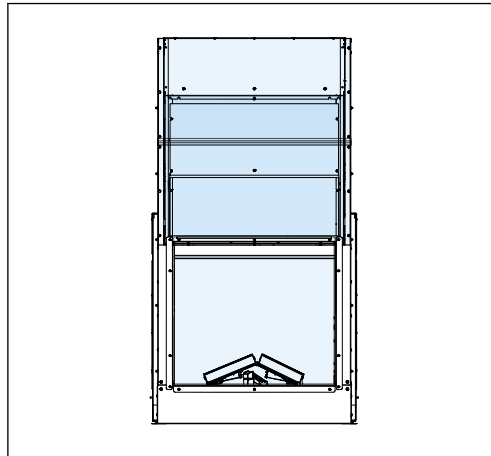
Abbildung 43. Kaminschirm in der Serviceposition
