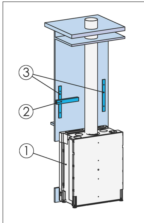
Abbildung 34. Installation eines Fernsehers über dem Gerät (Rückansicht)
