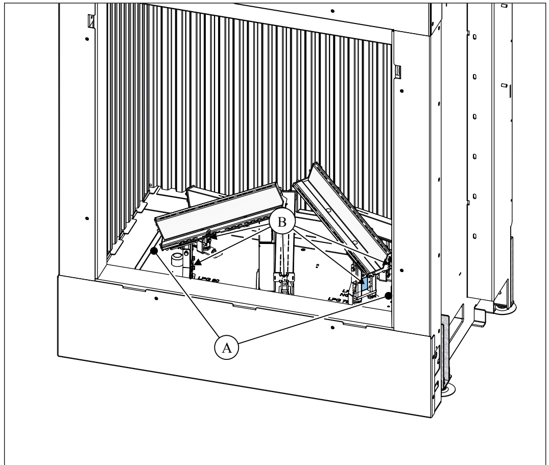
Abbildung 42. Positionen der Lufteinlass- und Primärlufteinlassöffnungen
