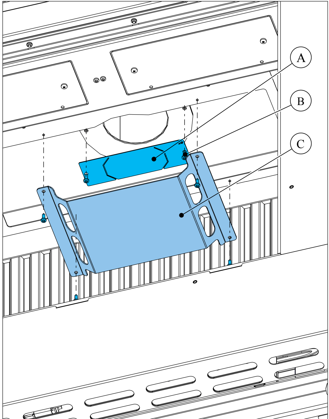
Abbildung 32. Begrenzerplatte und Umlenkplatte
