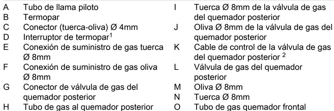
Figura 7. Conexiones del bloque regulador de gas
