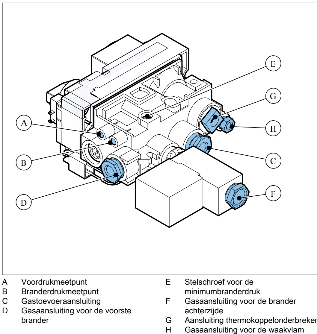
Figuur 5. Gasregelblok (achterzijde)
