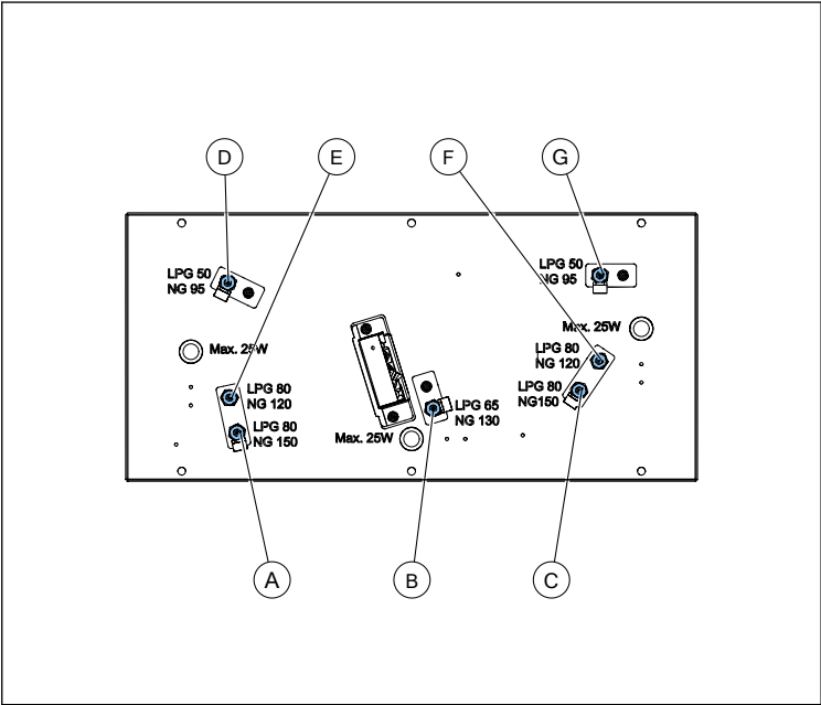
Abbildung 47. Positionen der Primrlufteinlsse und Gasinjektoren
